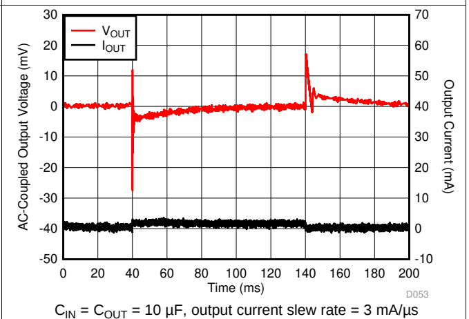
图 16. I_{OUT} Transient 3 μA to 3 mA
