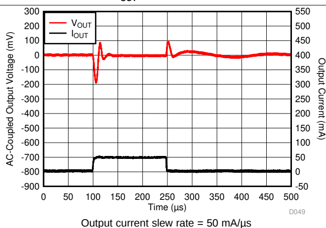
图 12. I_{OUT} Transient 1 mA to 50 mA
