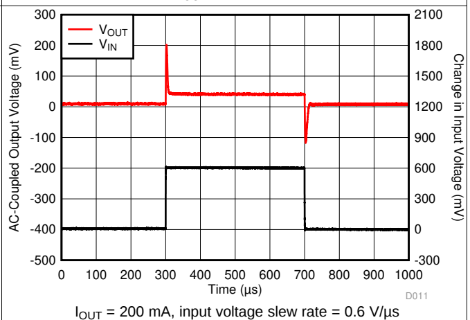
图 18. V_{IN} Transient
