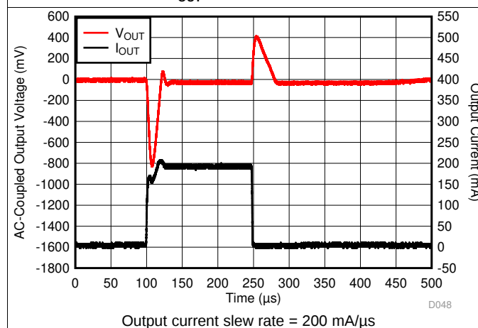
图 11. I_{OUT} Transient 0 mA to 200 mA
