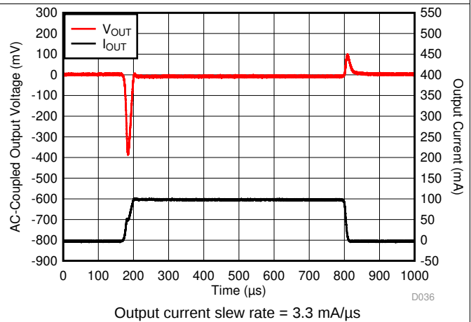
图 6. I_{OUT} Transient 0\text{ mA} to 100\text{ mA}
