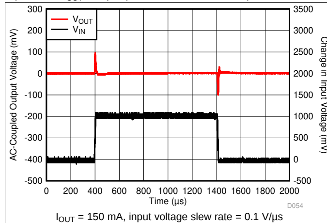
图 19. V_{IN} Transient
