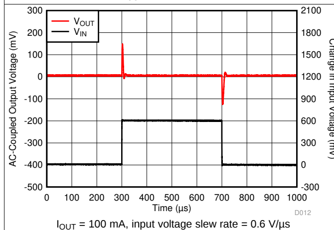
图 17. V_{IN} Transient
