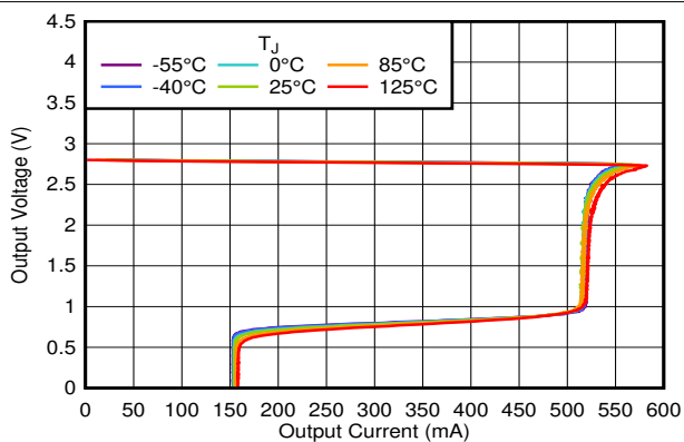
图 6-44. Current Limit
