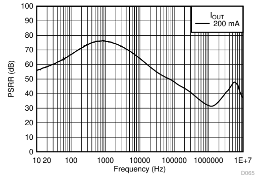
图 8-6. PSRR
