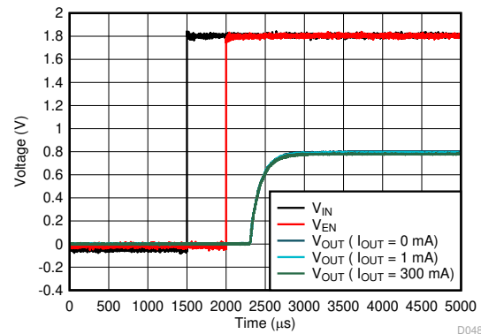
图 6-74. Start-Up
