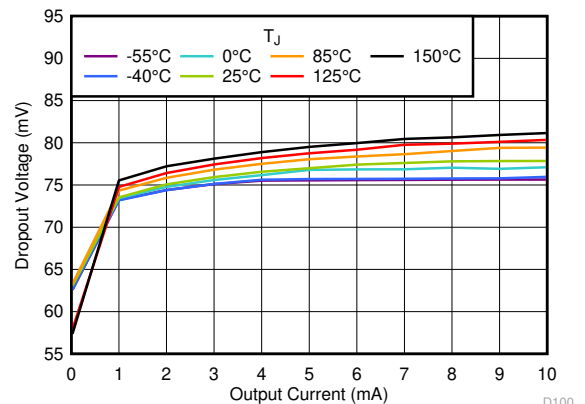
图 6-28. Dropout Voltage vs I_{OUT}
