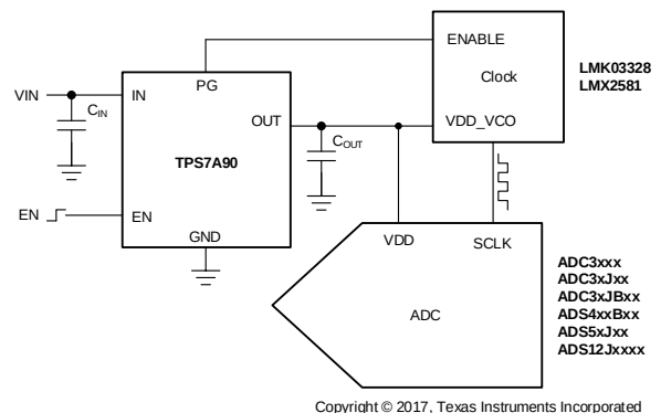
典型应用图
