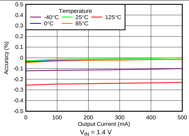
图 16. Load Regulation
