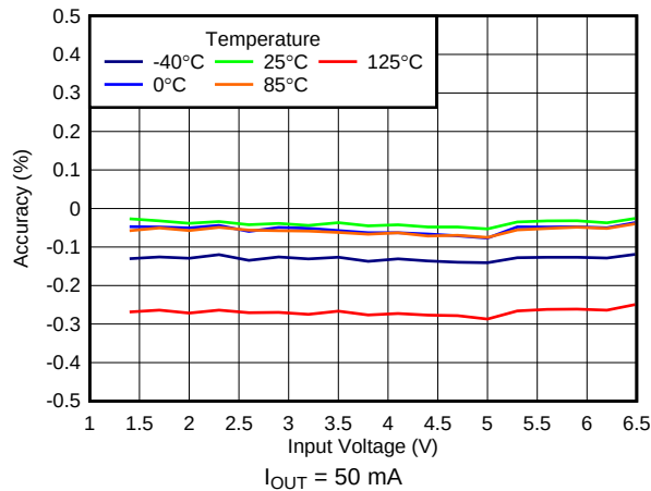
图 17. Line Regulation
