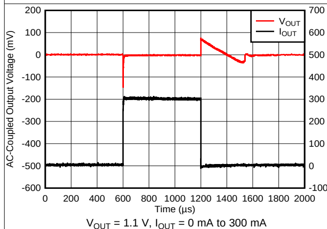
图 11. I_{OUT} Transient
