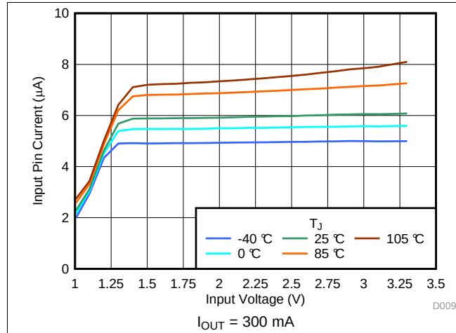
图 19. I_Q(V_{IN}) Over Temperature
