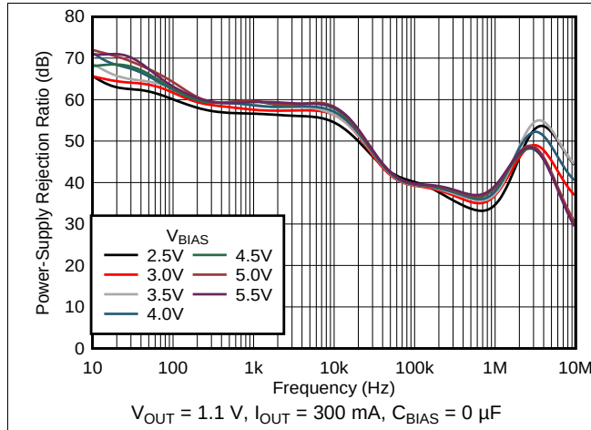
图 31. V_{BIAS} PSRR vs Frequency and V_{BIAS}
