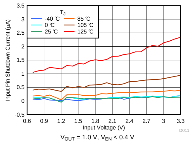
图 20. I_{SHDN}(V_{IN}) Over Temperature
