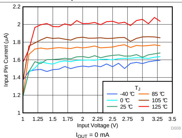
图 18. I_Q ( V_{IN} ) Over Temperature
