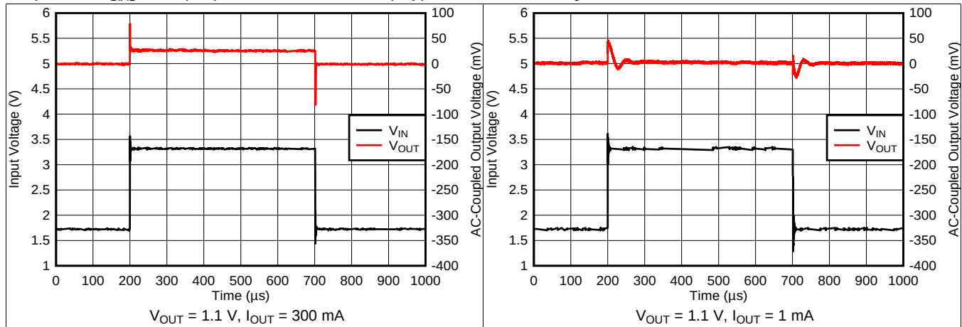
图 13. V_{IN} Transient
