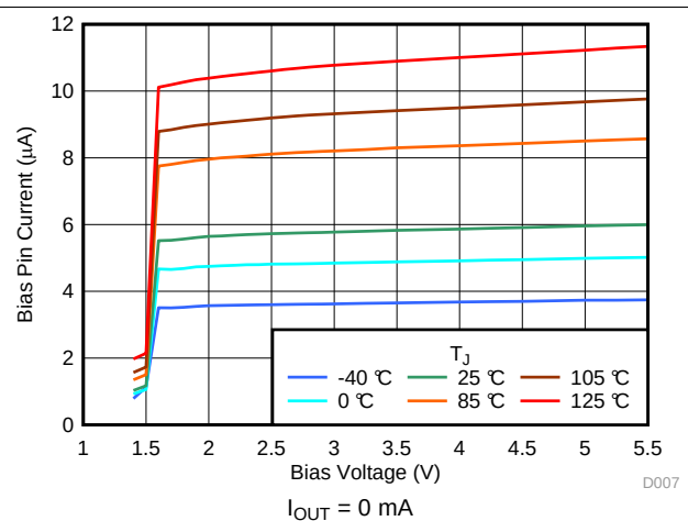
图 16. I_Q ( V_{BIAS} ) Over Temperature
