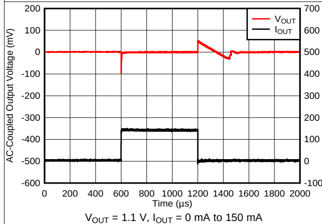
图 9. I_{OUT} Transient
