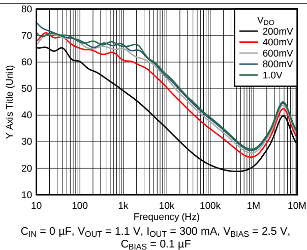
图 29. PSRR vs Frequency and V_{DO}
