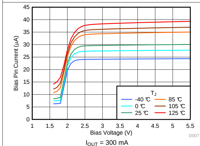
图 17. I_Q ( V_{BIAS} ) Over Temperature
