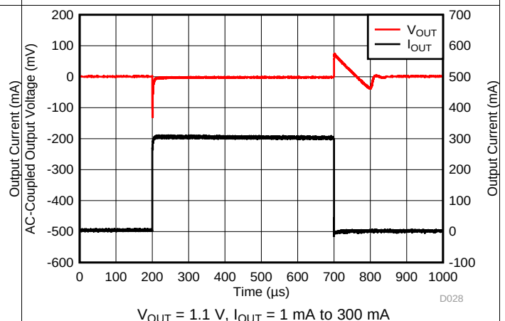
图 12. I_{OUT} Transient
