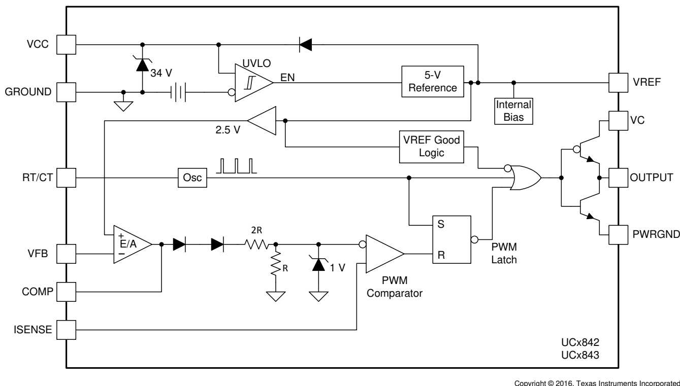
图 8-1. UCx842 和 UCx843 方框图 (不具有翻转触发器)
