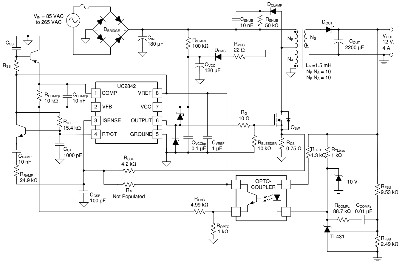
图 9-2. 典型应用设计示例原理图
