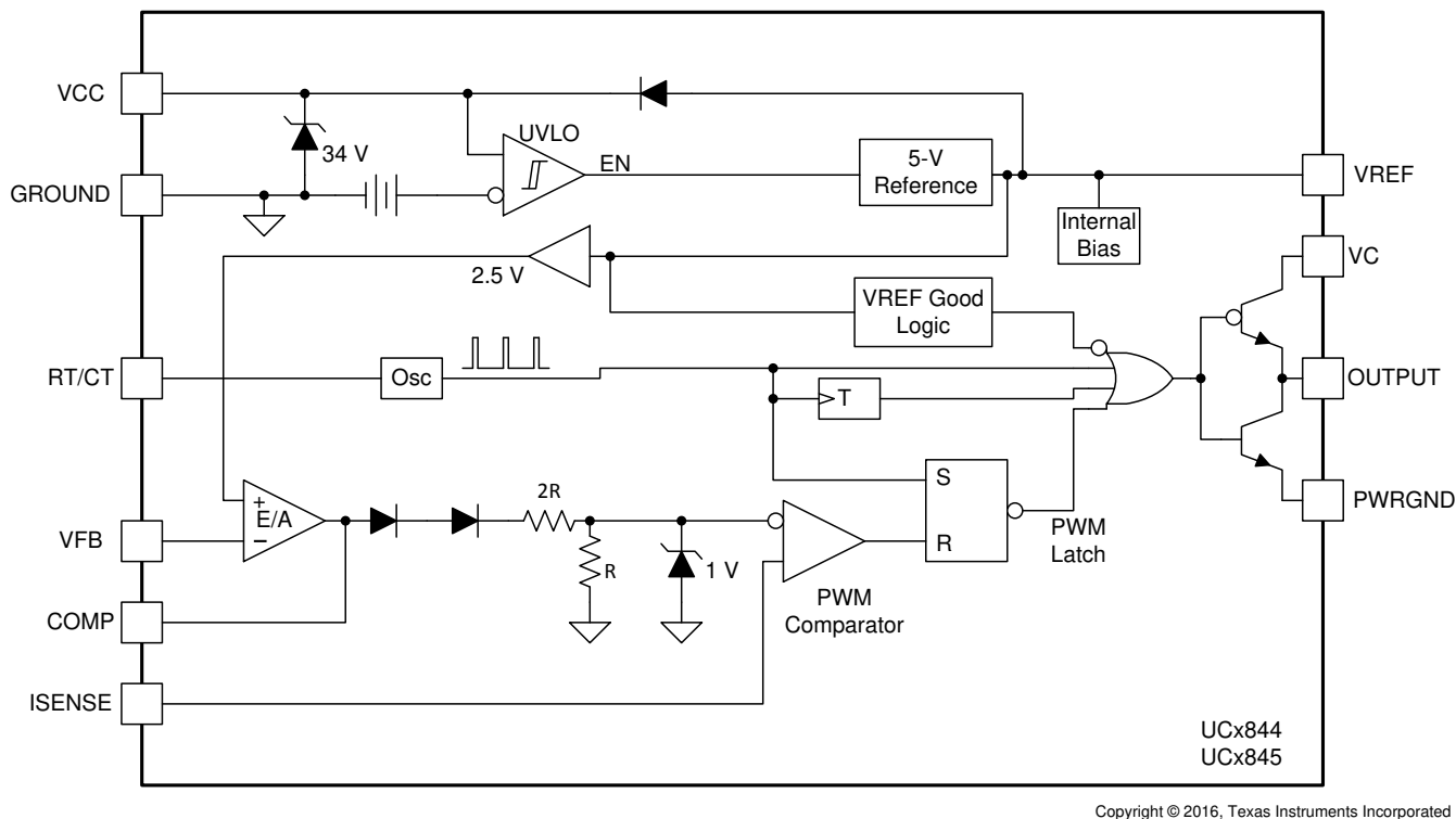
图 8-2. UCx844 和 UCx845 方框图 ( 具有翻转触发器 )
