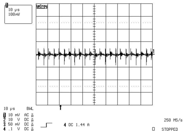
图 9-10. 满载条件下的输出电压纹波 (100mV/div)
