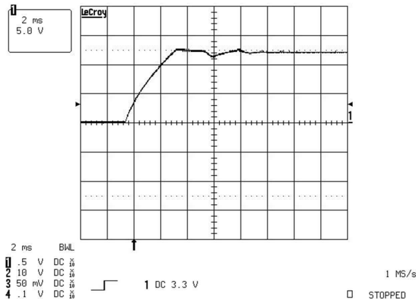
图 9-11. 满载启动条件下的输出电压行为 (5V/div)
