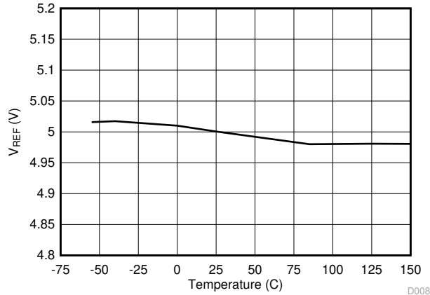
图 7-7. VREF 电压与温度间的关系
