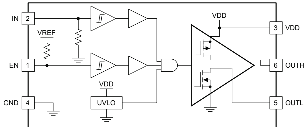
图 32. UCC27531
