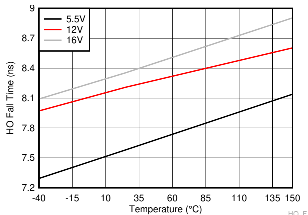
图 6-25. HO Fall Time
