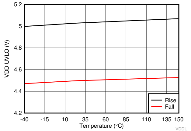
图 6-14. VDD UVLO Threshold
