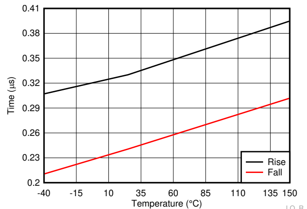
图 6-24. HO Rise Time
