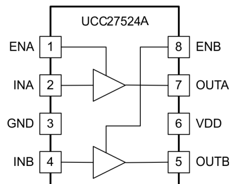
双路非反相输入
