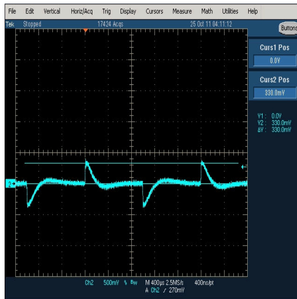
1A-16A-1A Vin =385V 图 10-10. Load Transient
