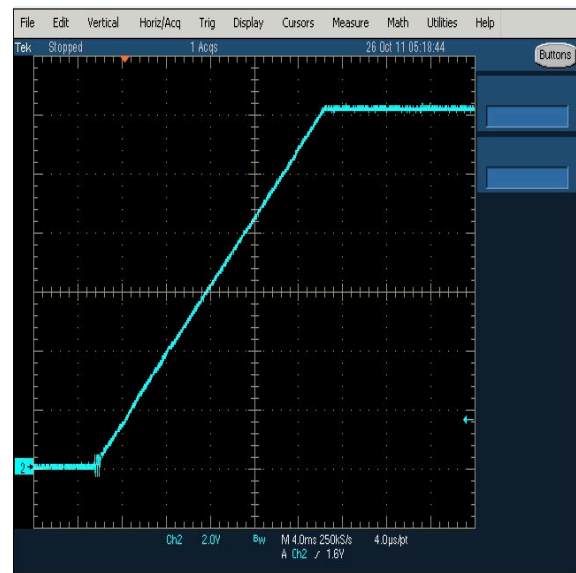
30A Load syncFETs off 图 10-11. V OUT Soft Start
