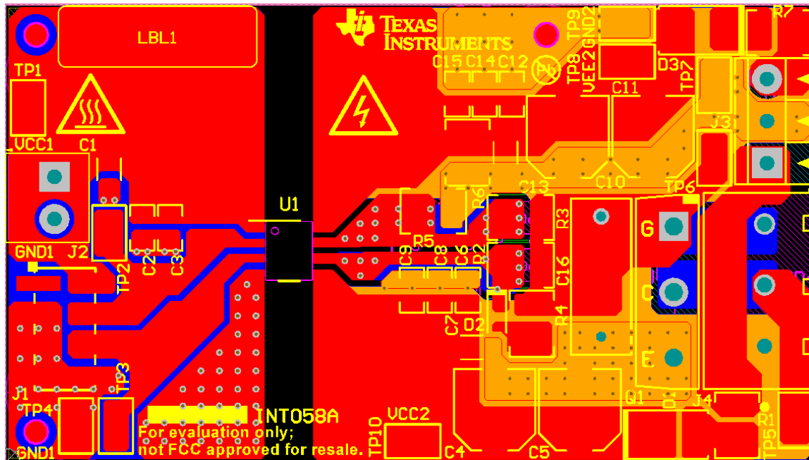
图 63. Layout Example
