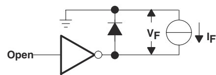
图 7-8. V_F 测试电路
