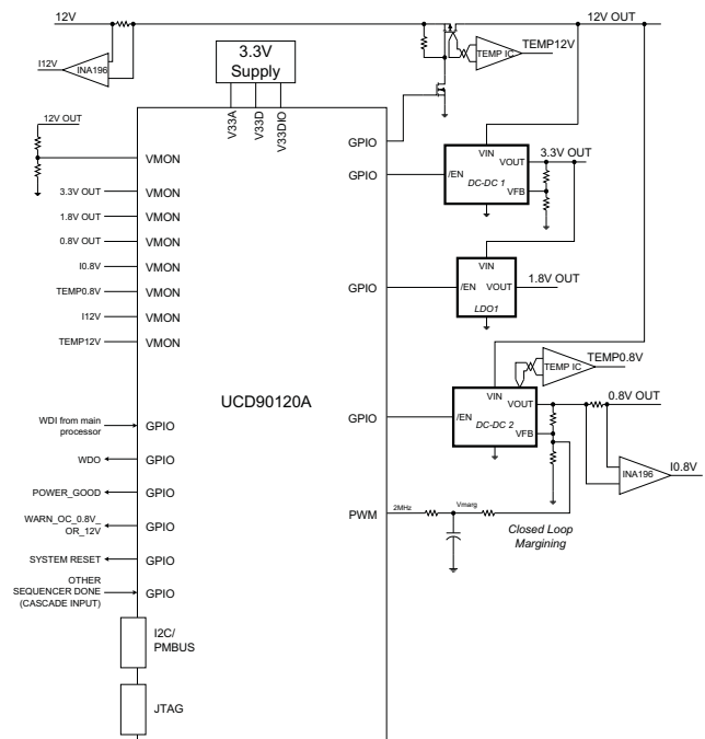
简化原理图
