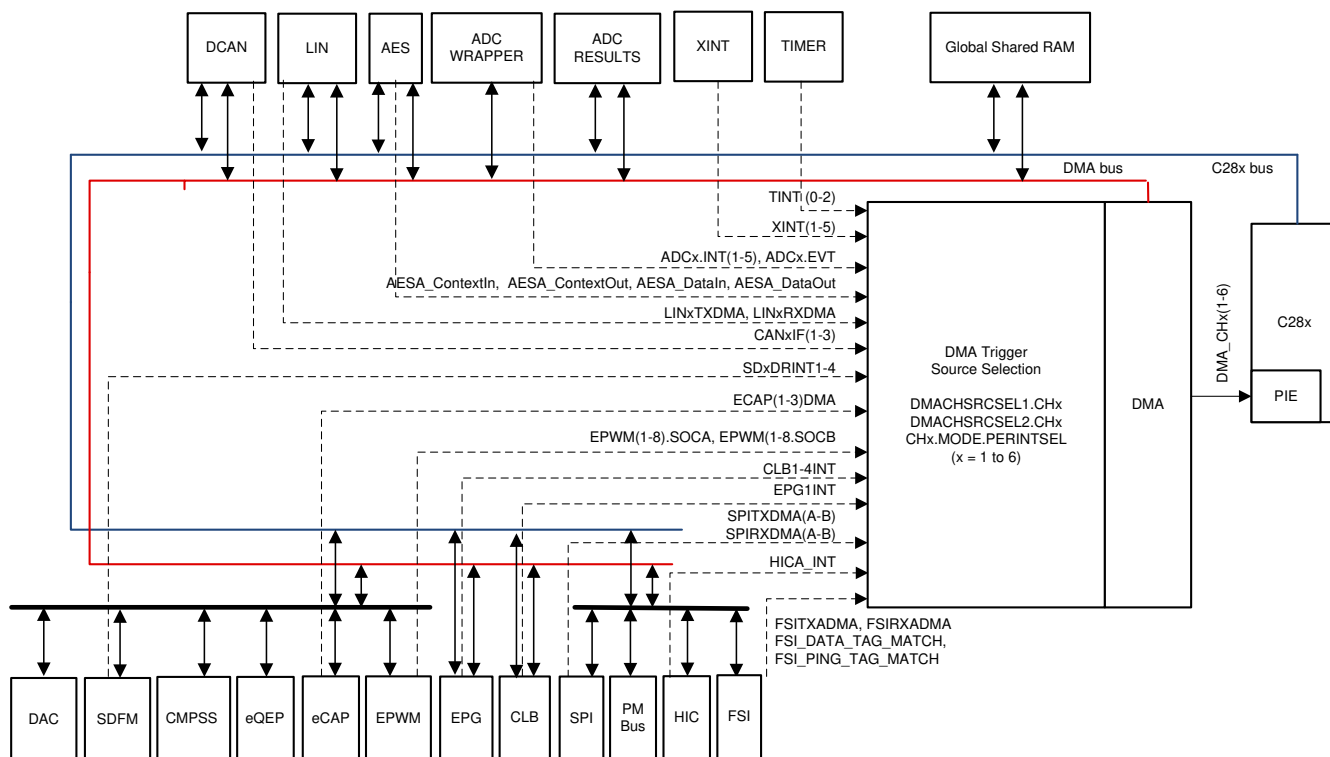
图 7-3. DMA 方框图
