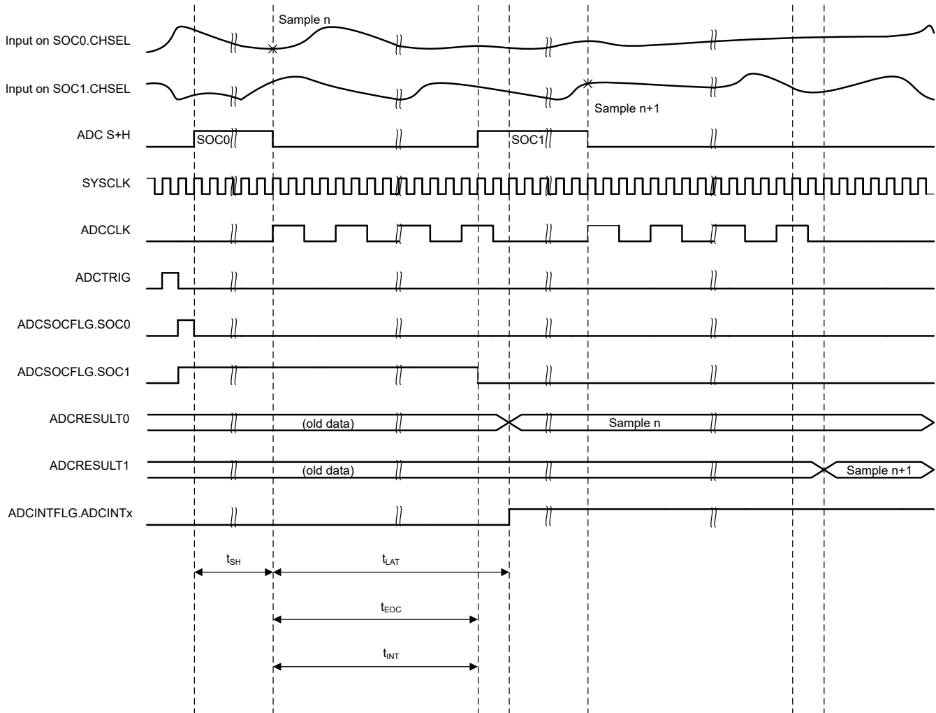
图 6-40. ADC 时序
