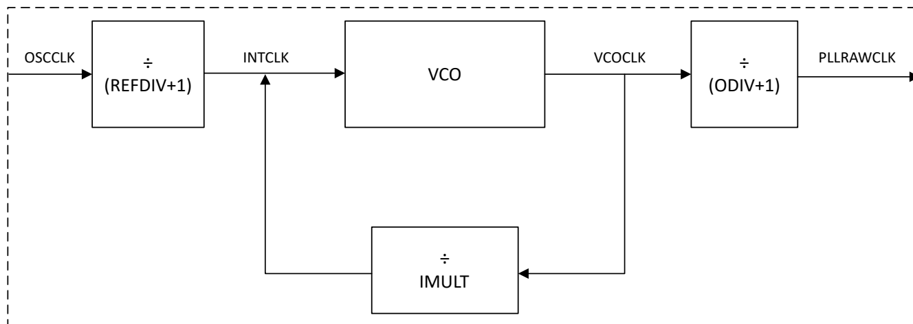
图 6-10. 系统 PLL
