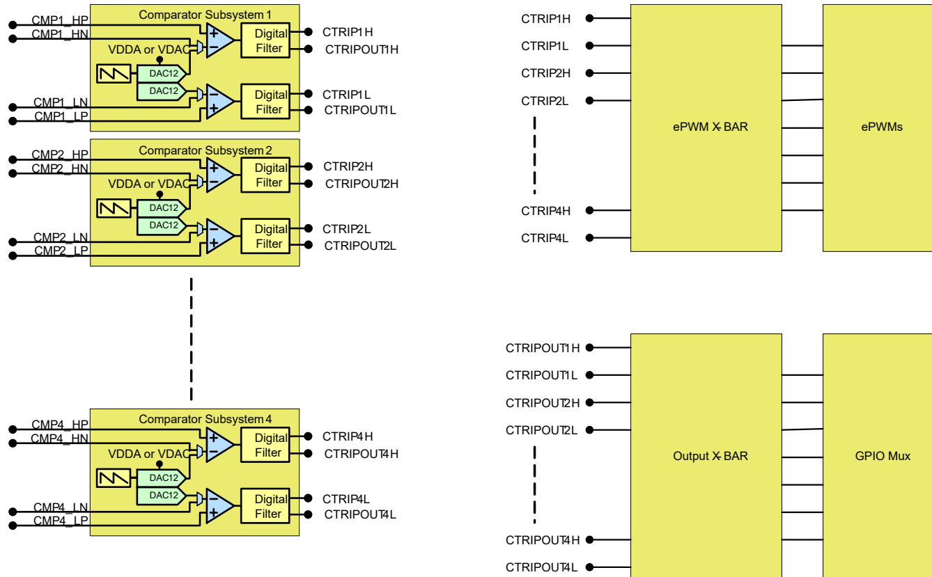
图 6-41. CMPSS 连接
