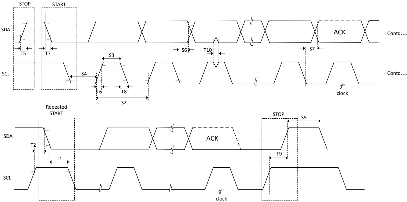
图 6-62. I2C 时序图
