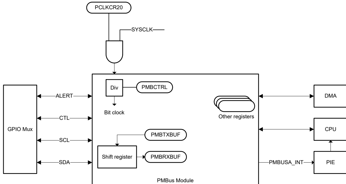
图 6-63. PMBus 方框图
