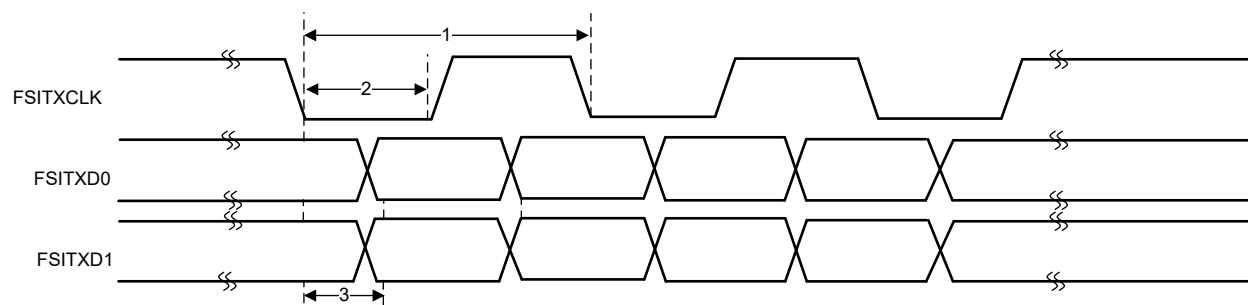
图 6-73. FSITX 时序
