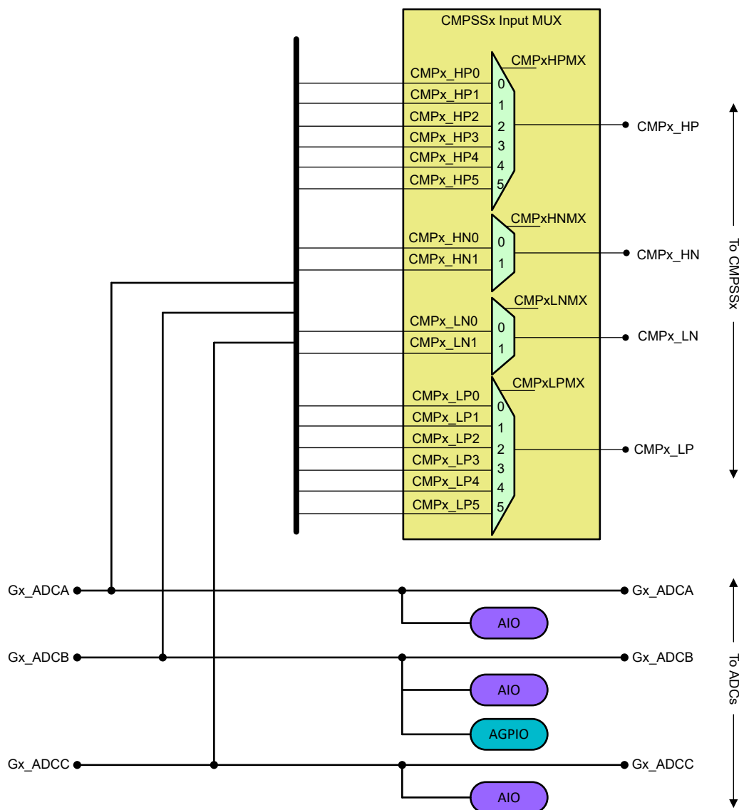
图 6-36. 模拟组连接
