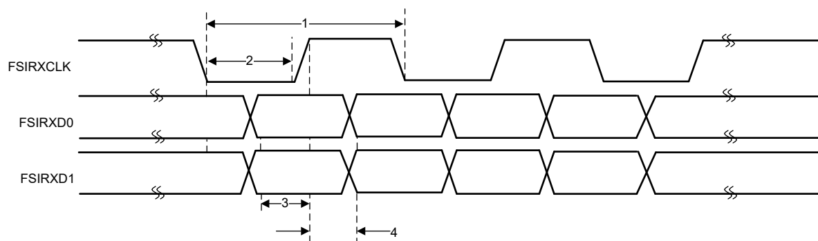
图 6-76. FSIRX 时序
