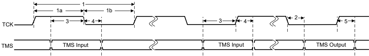
图 6-23. cJTAG 时序
