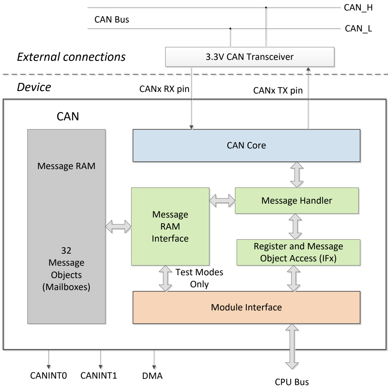
图 6-59. CAN 方框图
