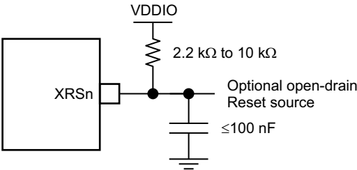
图 6-6. 复位电路
