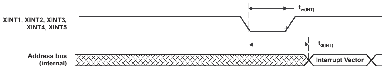
图 6-28. 外部中断时序
