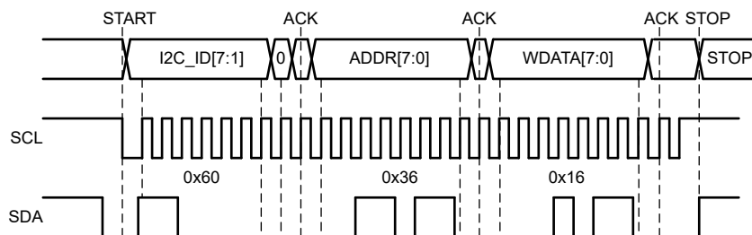
图 7-8. I²C Write Cycle without CRC
