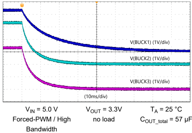
图 8-15. Buck Discharge
