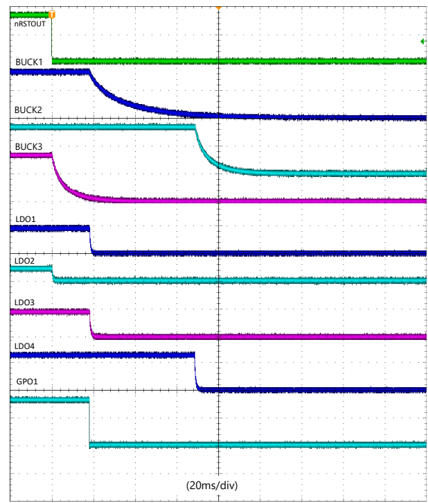
图 8-16. LDOs Discharge
