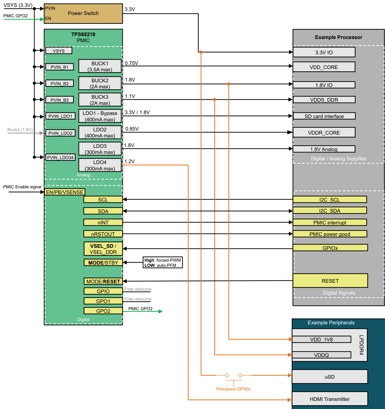
图 8-1. Example Power Map
