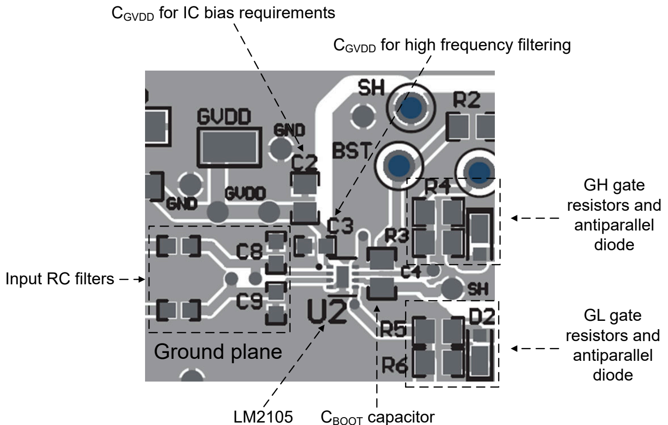
图 10-1. Layout Example
