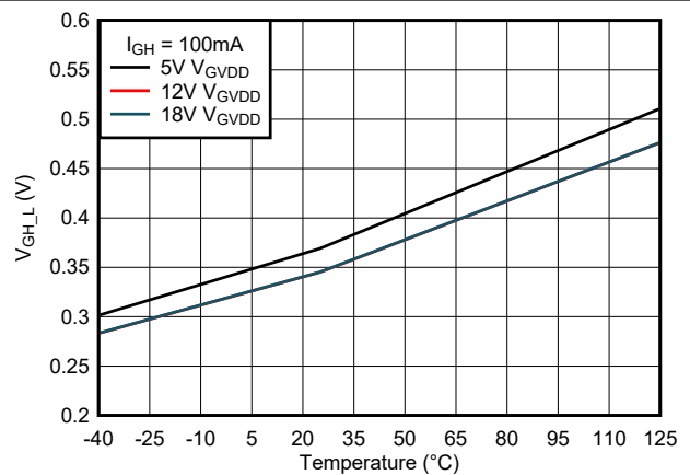
图 6-11. GH Output Low Voltage vs Temperature
