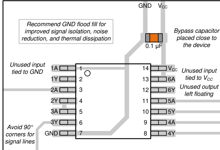
图 9-3. 采用 PW 封装的 SN74LV14B-EP 布局示例
