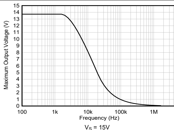
图 6-32. 最大输出电压与频率间的关系 V_S = 15\text{V}
