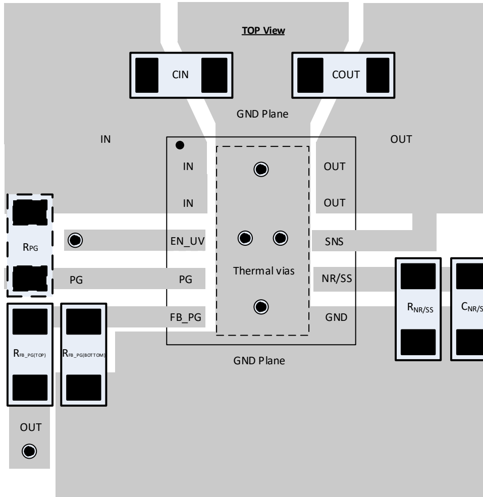
图 8-33. Example Layout
