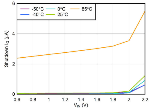
图 6-8. V_{\text{IN}} Shutdown I_Q vs V_{\text{IN}}
