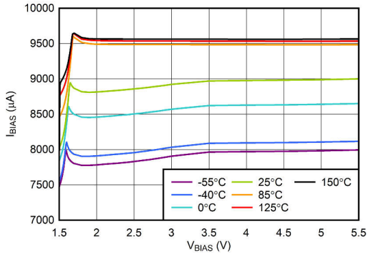
图 6-7. V_{\text{BIAS}} Input Current vs V_{\text{BIAS}}
