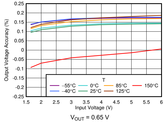
图 6-2. Output Accuracy vs V_{IN}
