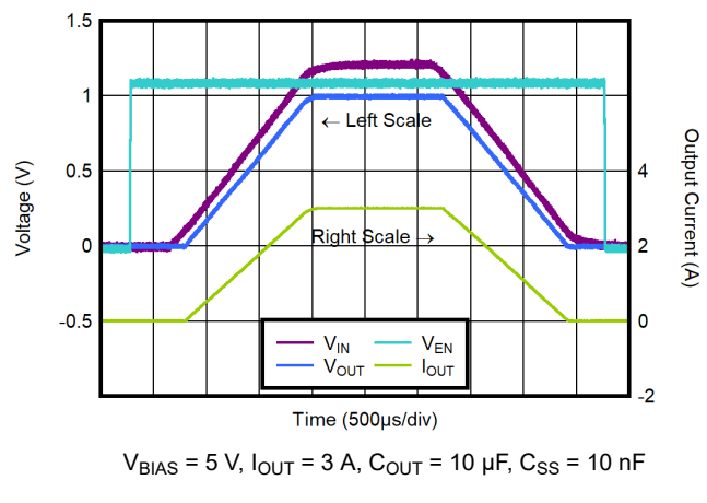
图 6-18. Input Ramp Response
