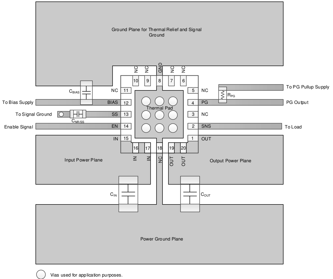
图 8-5. Example Layout
