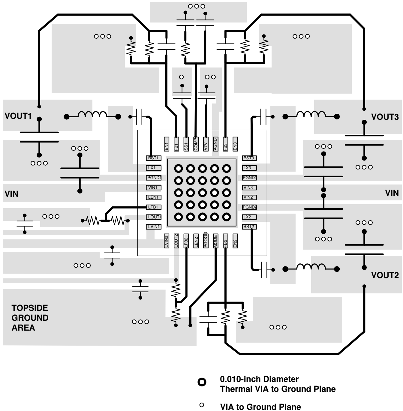
图 8-37. PCB Layout
