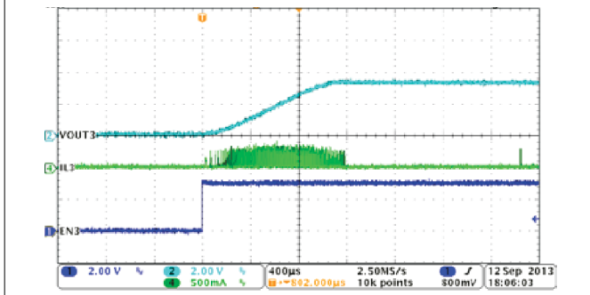
图 8-7. PSM Mode Buck3, Soft-Start With No Load
