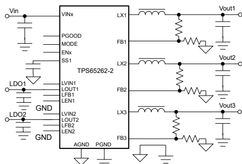
应用原理图
