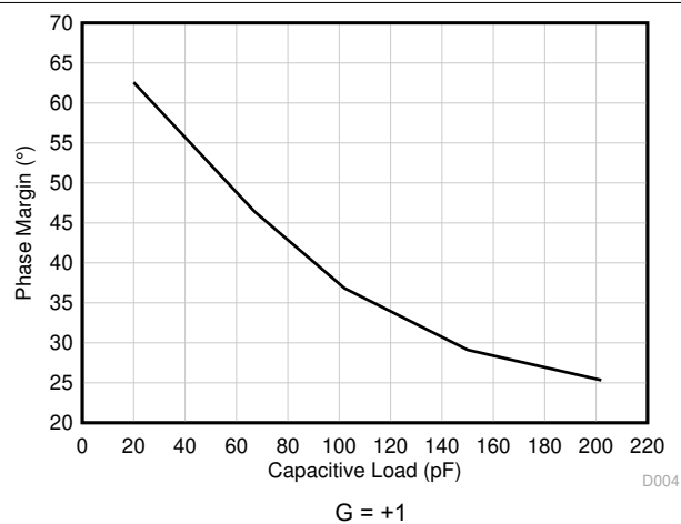
图 6-33. Phase Margin vs Capacitive Load
