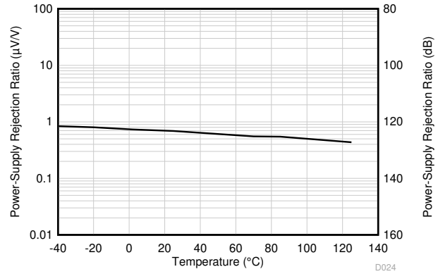
图 6-24. PSRR vs Temperature
