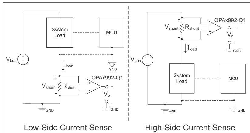
OPAx992-Q1 在电流检测应用中
