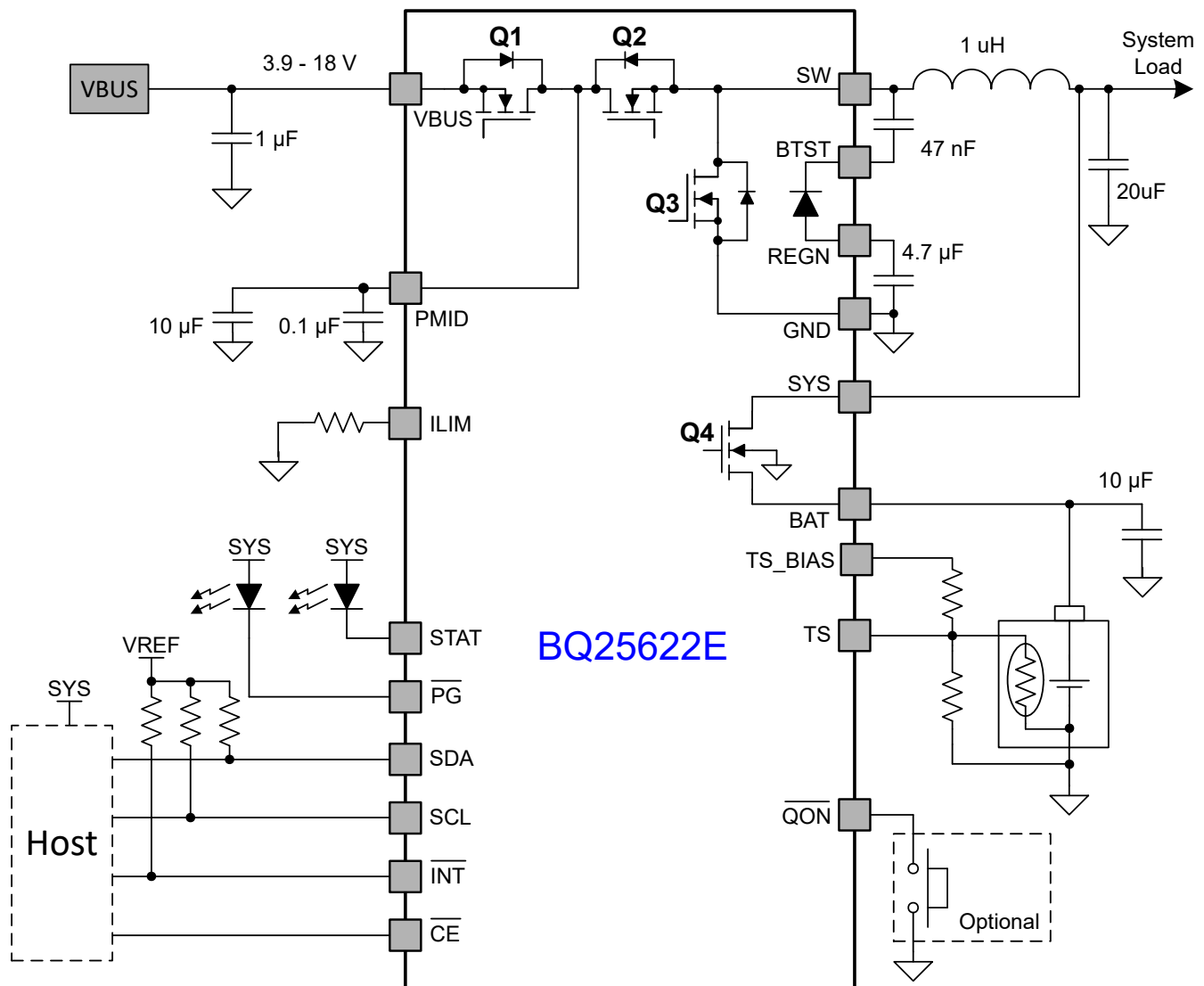
图 10-1. BQ25622E 应用示意图
