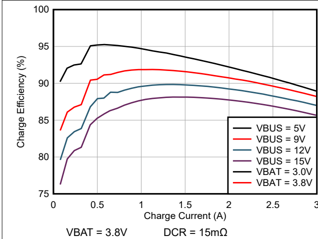
图 8-1. 充电效率与充电电流间的关系
