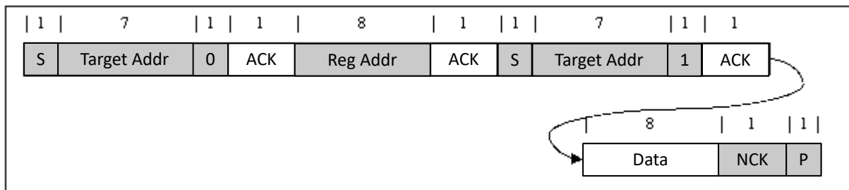
图 9-11. 单次读取
