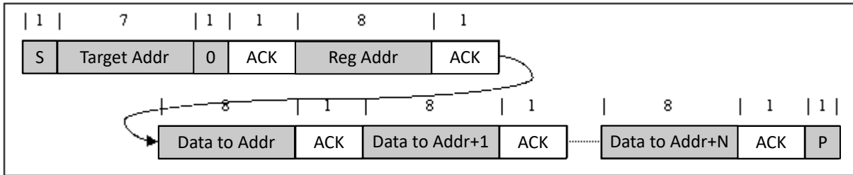
图 9-12. 多重写入
