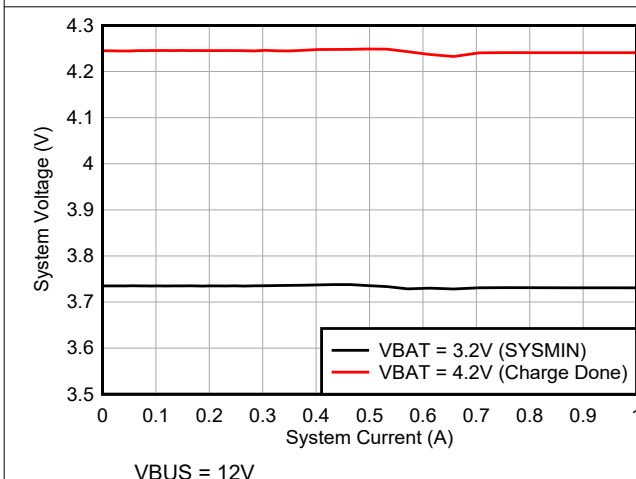
图 8-5. SYSMIN 和充电完成后的系统负载调节
