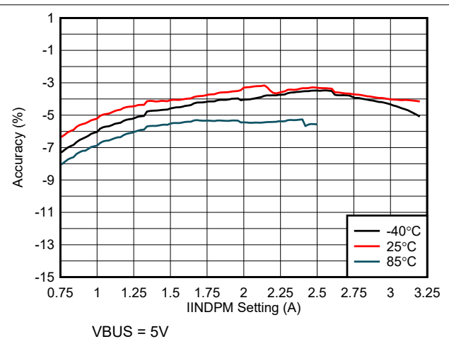
图 8-6. 输入电流调节精度与 IINDPM 设置间的关系
