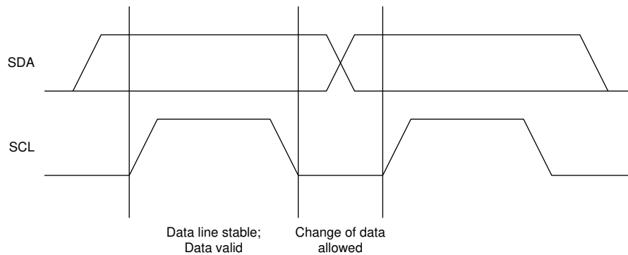
图 9-6. 在 I 2 C 总线上的位传输
