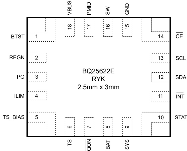
图 7-1. BQ25622E 引脚排列，18 引脚 WQFN 顶视图
