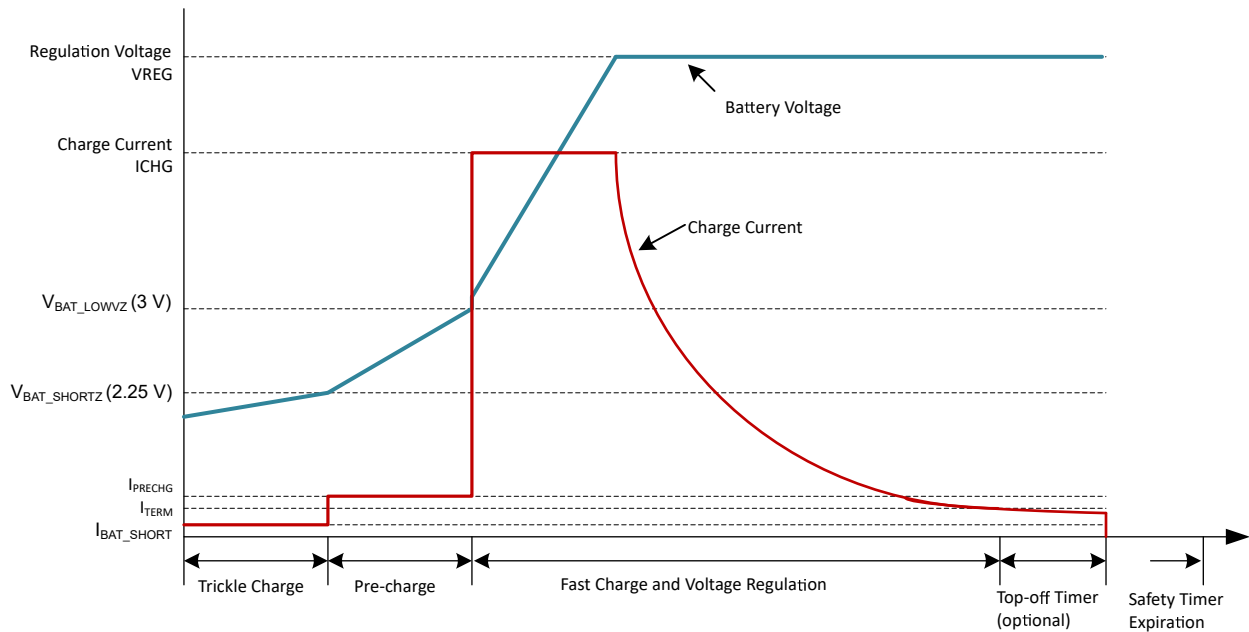
图 9-1. 电池充电曲线
