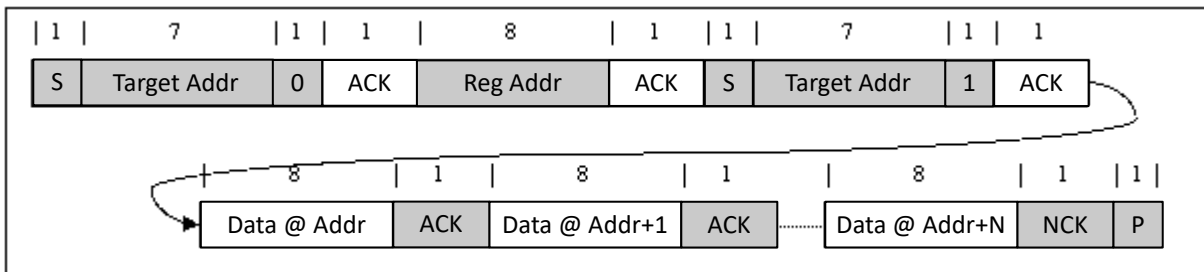
图 9-13. 多重读取
