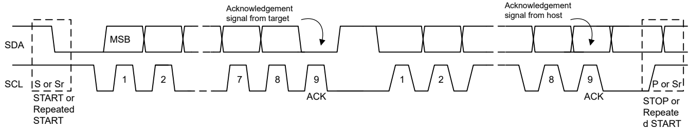
图 9-8. I 2 C 总线上的数据传输
