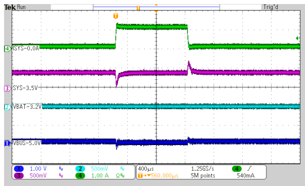
图 10-8. 降压模式下的 PFM 开关
