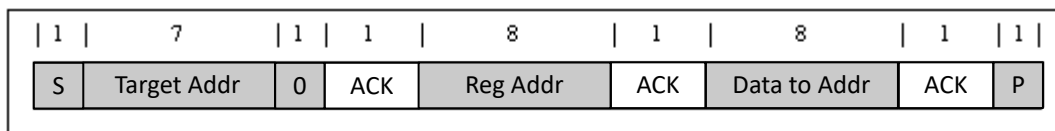
图 9-10. 单独写入
