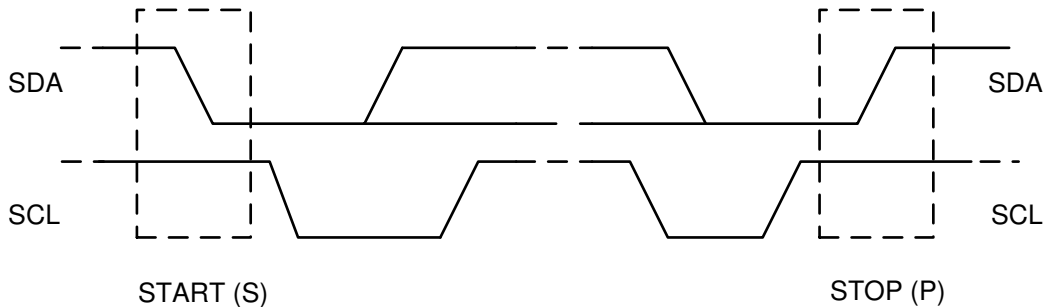
图 9-7. I 2 C 总线上的 START 和 STOP 条件
