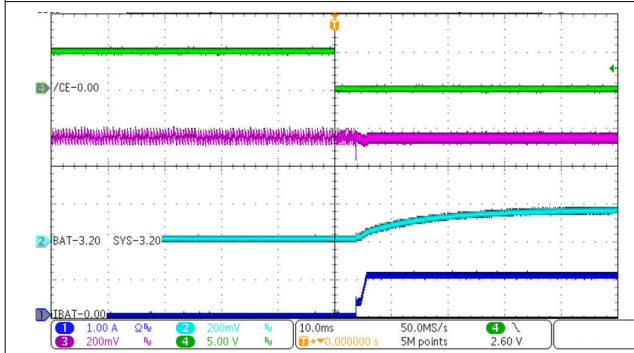
图 10-2. 在充电启用时上电
