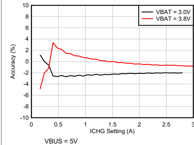
图 8-3. 充电电流精度与 ICHG 设置间的关系
