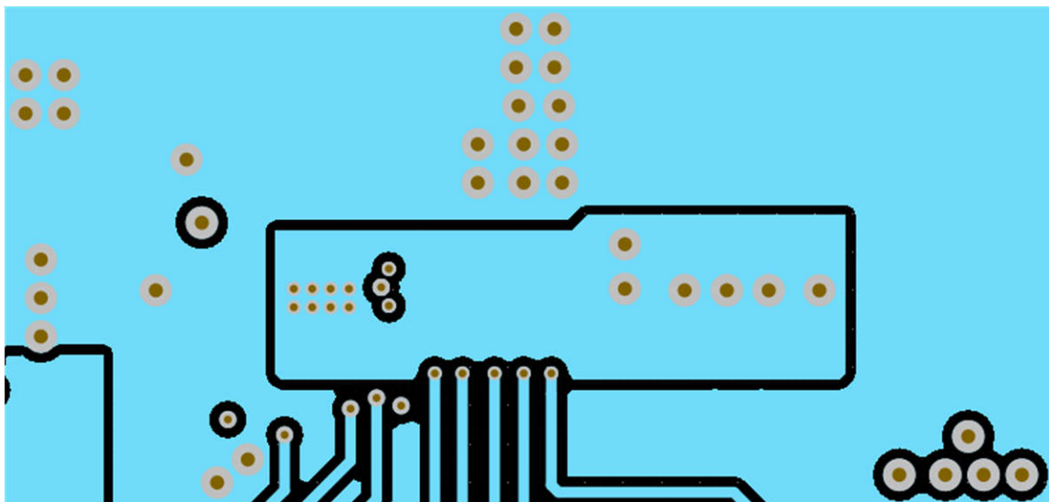
图 12-3. 布局示例：内层 3（AGND 覆铜；SW 节点覆铜；信号布线）
