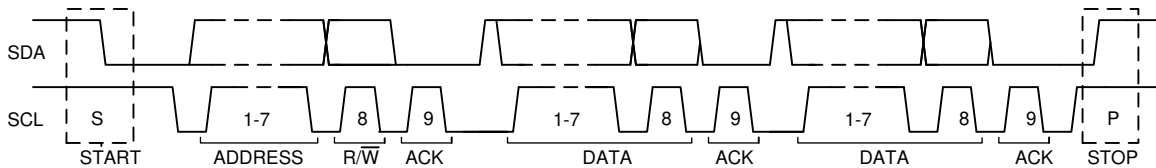
图 9-9. I 2 C 总线上的完整数据传输
