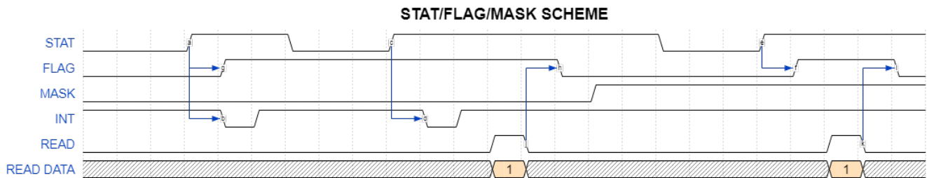
图 9-3. STAT、FLAG、和 MASK 之间的关系
