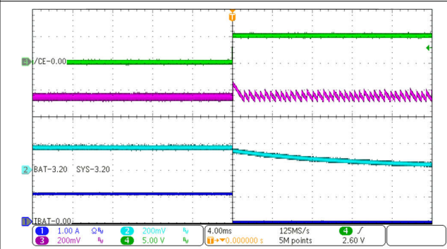
图 10-3. 断电
