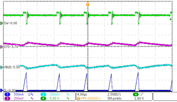
图 10-8. 降压模式下的 PFM 开关
