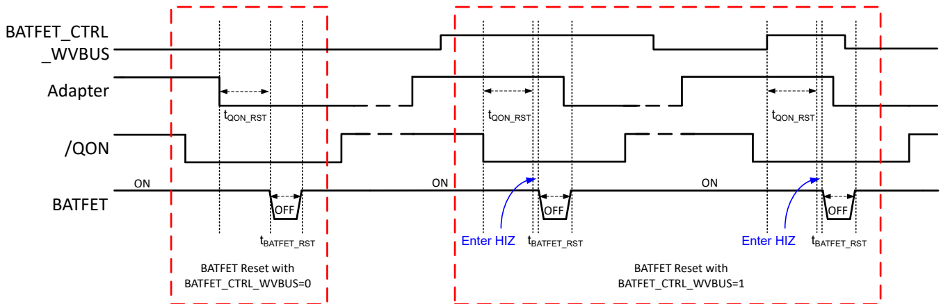
图 9-4. 系统电源复位时序
