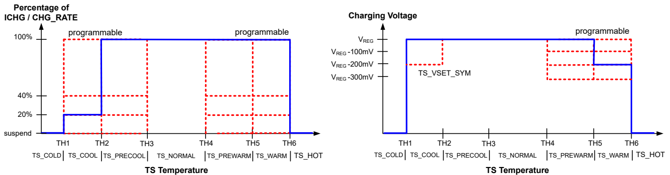
图 9-2. TS 充电值
