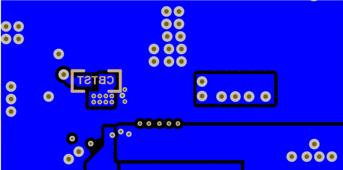
图 12-4. 布局示例：来自顶部的底层 X 射线 ( PGND 覆铜；BTST 电容器；冗余 SW、SYS 和 BAT 覆铜 )
