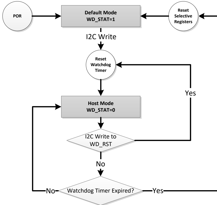
图 9-5. 看门狗计时器流程图
