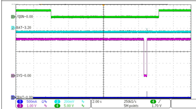
图 10-4. 充电启用
