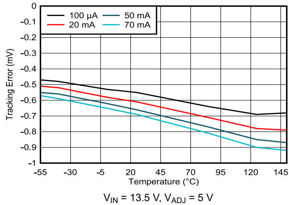
图 6-1. Tracking Error vs Ambient Temperature
