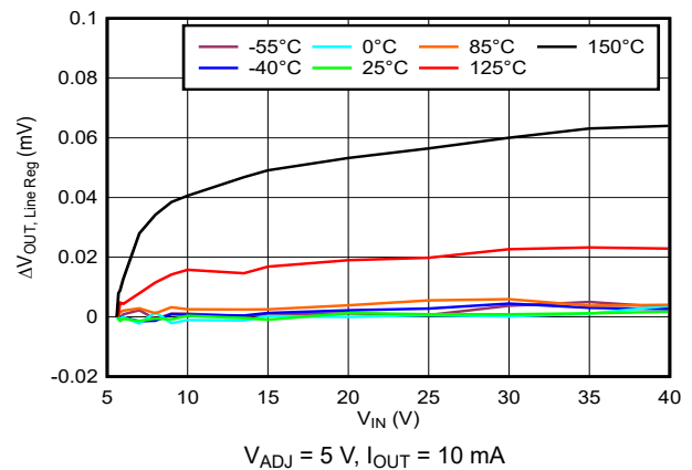
图 6-4. Line Regulation
