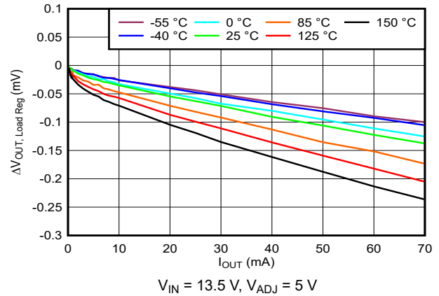
图 6-2. Load Regulation
