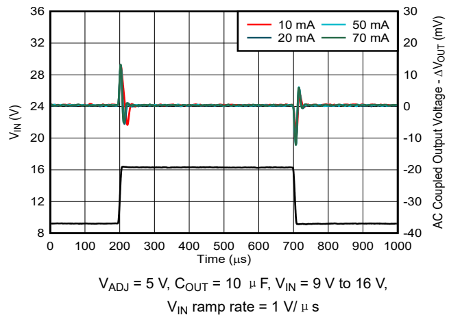
图 6-18. Line Transient
