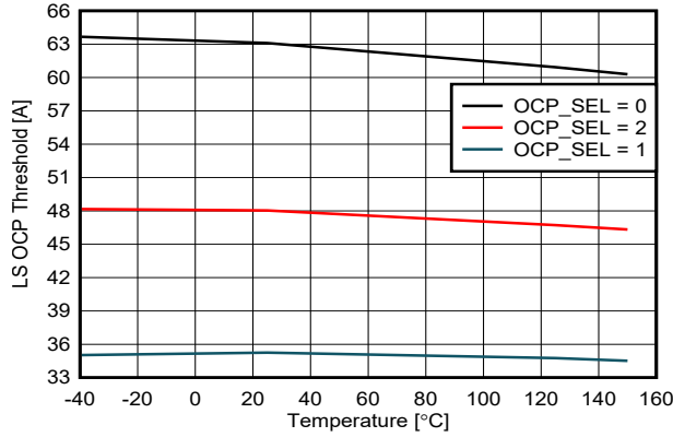
图 7-12. LS OCP 阈值与温度之间的关系 ( V_{VM} = 13.5V )
