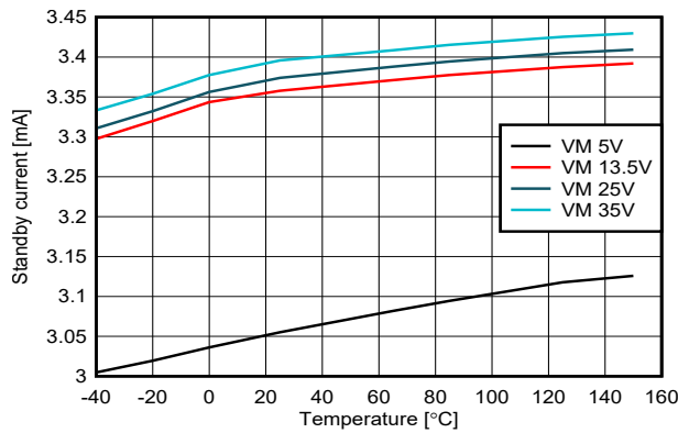
图 7-14. 待机状态下 VM 上的电流与温度之间的关系
