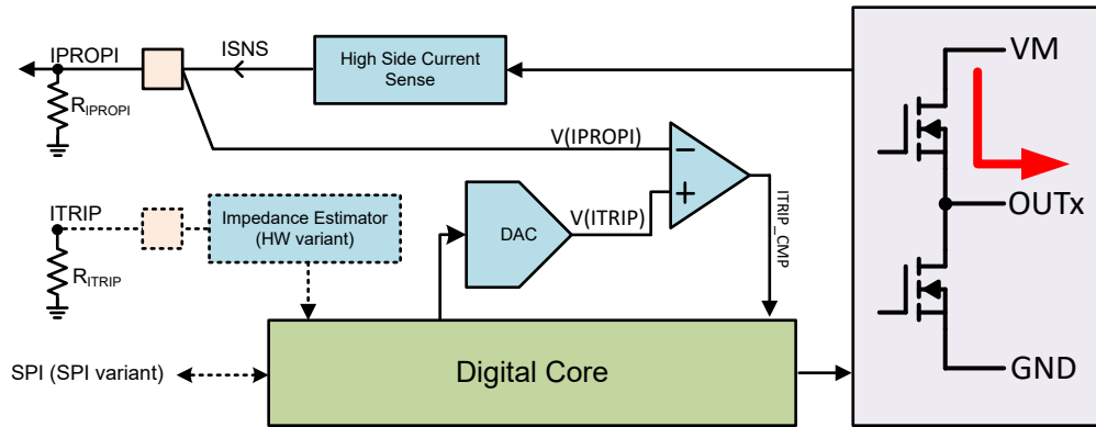
图 8-3. ITRIP 实现
