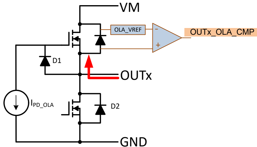
图 8-6. 导通状态诊断
