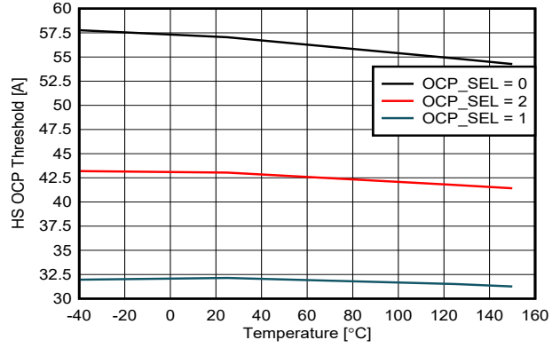
图 7-13. HS OCP 阈值与温度之间的关系 ( V_{VM} = 13.5V )
