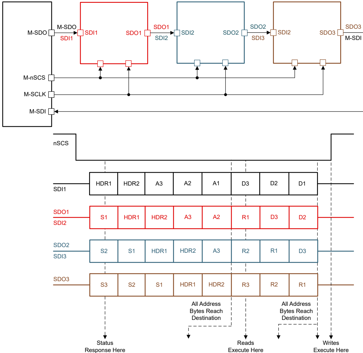
图 8-12. 菊花链 SPI 操作
