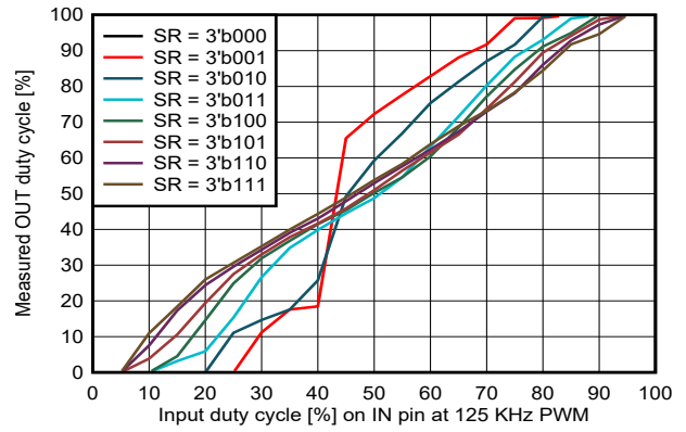
图 7-19. 用于 HS 再循环的 V_{VM} = 13.5V 时，PWM 频率为 125 KHz 时测得的占空比与输入占空比之间的关系
