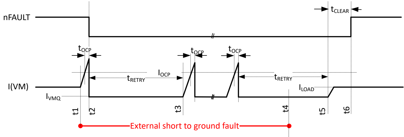
图 7-8. 采用重试 (RETRY) 设置的故障反应 (当 OUT 接地短路时, 针对在高侧发生的 OCP 显示)
