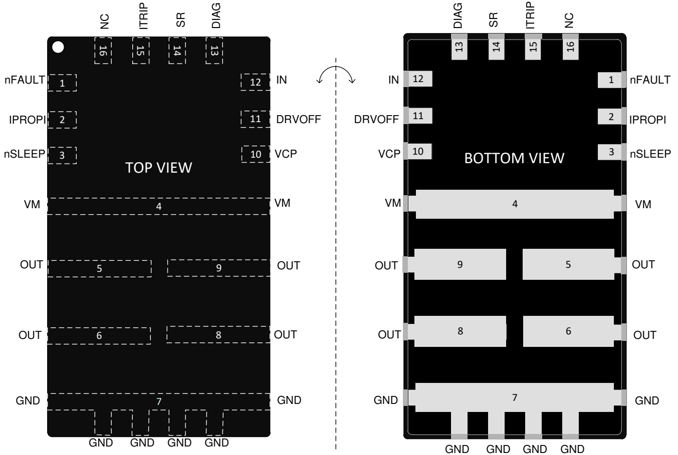
图 6-1. 采用 VQFN-HR (16) 封装的 DRV8144H-Q1 HW 型号
