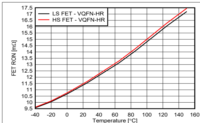
图 7-10. V_{VM} = 13.5V 时 R_{HS\_ON} 和 R_{LS\_ON} 与温度之间的关系
