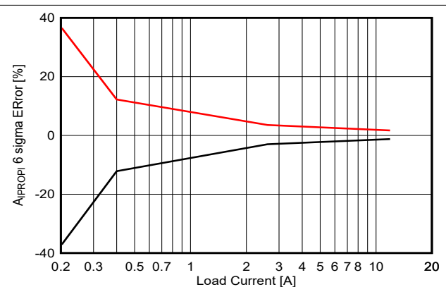
图 7-11. V_{VM} = 13.5V 时 A_{IPROPI} 增益误差与 V 负载电流之间的关系
