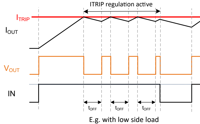
图 8-4. 固定 TOFF ITRIP 电流调节
