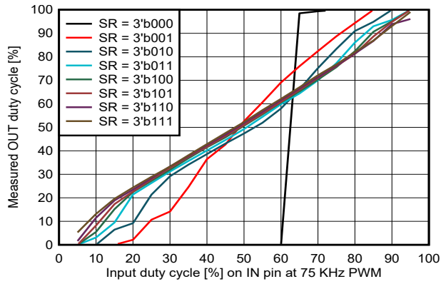
图 7-18. 用于 HS 再循环的 V_{VM} = 13.5V 时，PWM 频率为 75 KHz 时测得的占空比与输入占空比之间的关系
