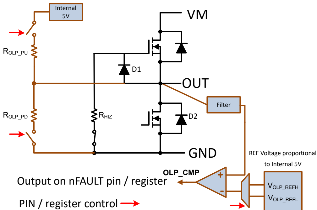
图 8-5. 关闭状态 (无源) 诊断
