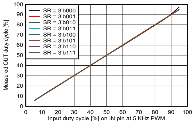
图 7-16. 用于 HS 再循环的 V_{VM} = 13.5V 时, PWM 频率为 5KHz 时测得的占空比与输入占空比之间的关系
