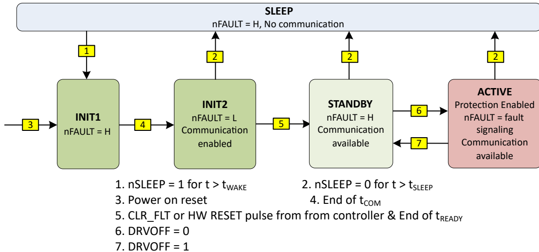
图 8-7. 说明性状态图
