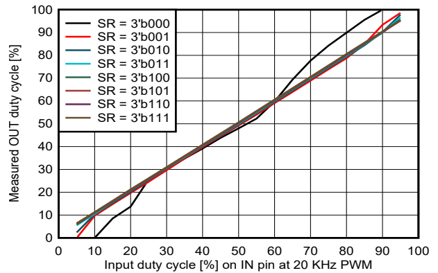
图 7-17. 用于 HS 再循环的 V_{VM} = 13.5V 时, PWM 频率为 20 KHz 时测得的占空比与输入占空比之间的关系
