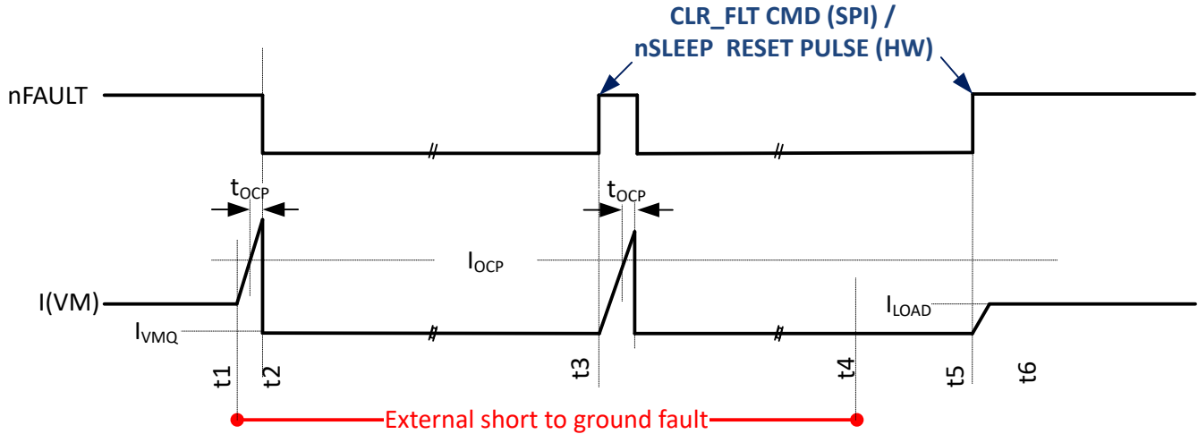
图 7-9. 采用锁存 ( Latch ) 设置的故障反应 ( 当 OUT 接地短路时, 针对在高侧发生的 OCP 显示 )
