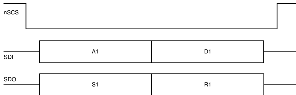
图 8-9. SPI 数据 - 标准“16 位”帧
