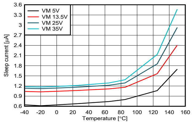
图 7-15. 休眠状态下 VM 上的电流与温度之间的关系
