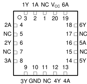
图 5-3. SN54AHCT04 FK Package, 20-Pin (Top View)
