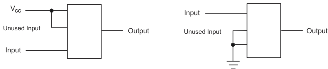
图 9-4. Layout Diagram
