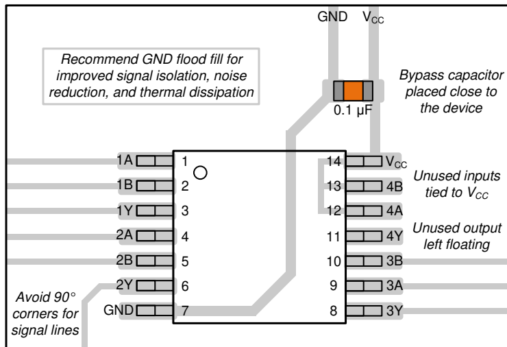
图 11-1. SN74LV6T17 的示例布局
