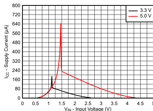
图 7-2. 3.3V 和 5.0V 输入电压电源上的电源电流
