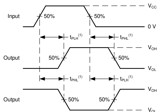
图 8-2. 电压波形传播延迟
