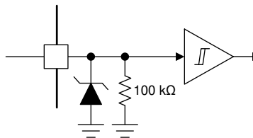
图 9-9. 逻辑电平输入
