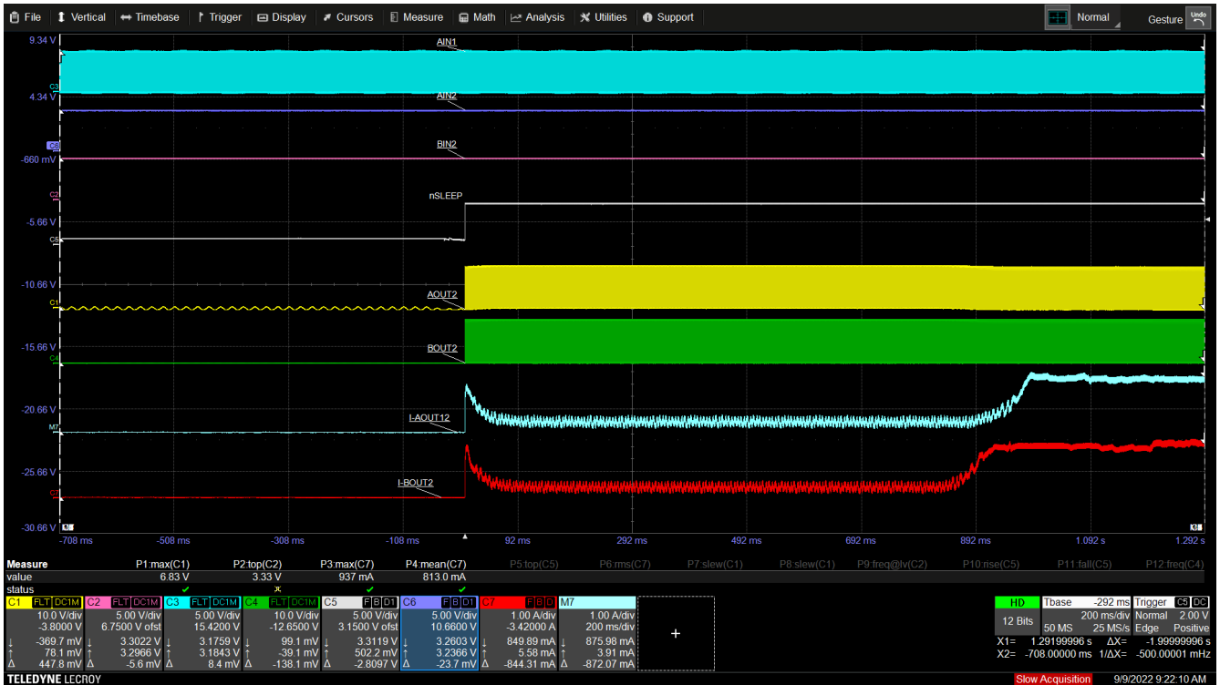
图 10-9. 无电流调节
