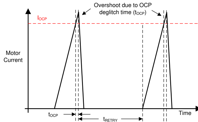
图 9-6. OCP 运行
