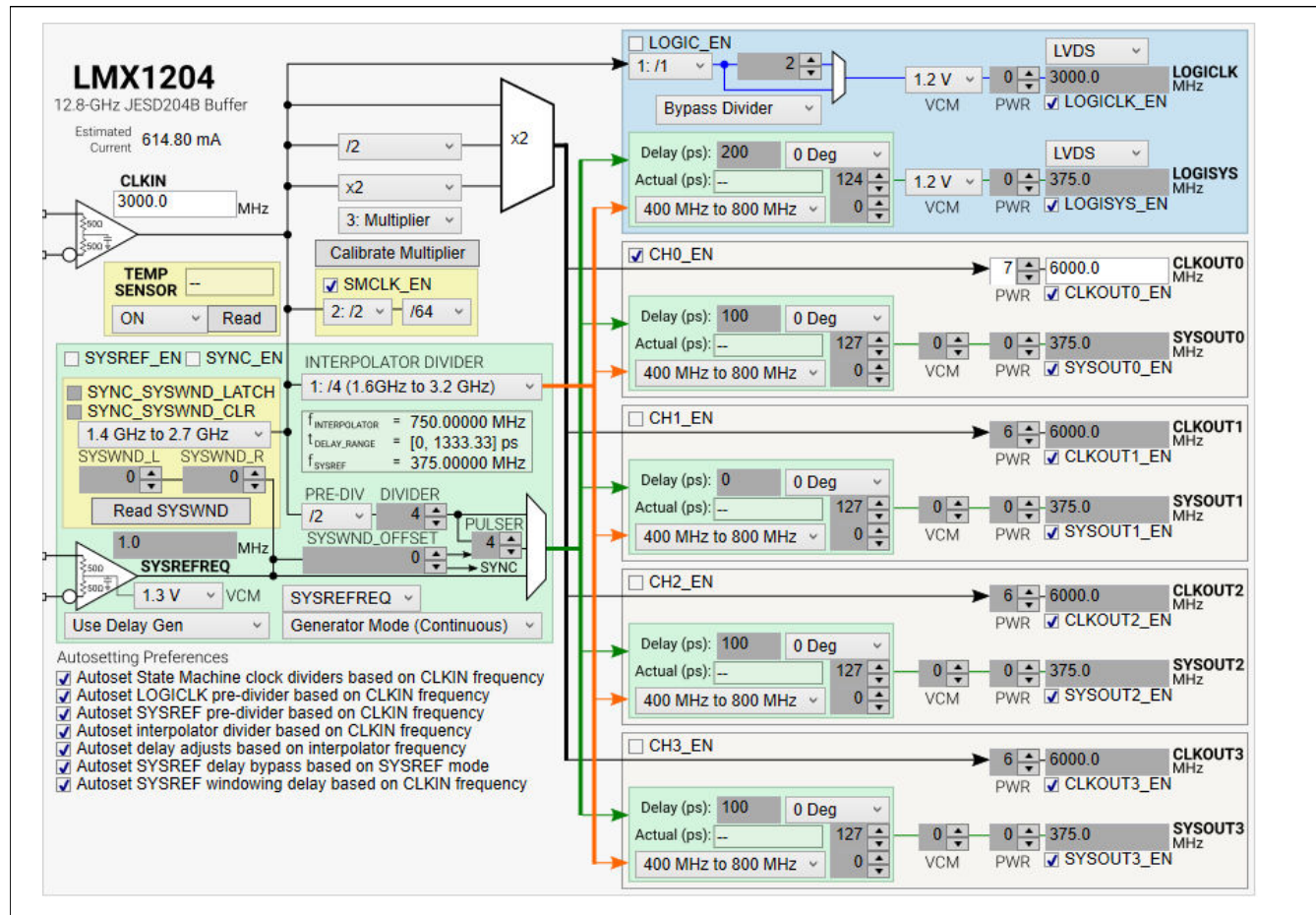
图 8-2. LMX1204 TICS Pro Setup
