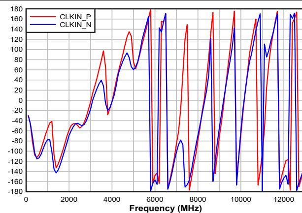
图 6-31. CLKIN S11 Phase
