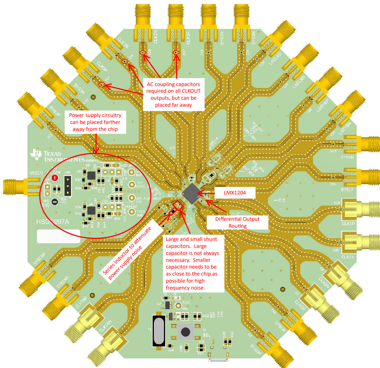
图 8-4. Layout Example
