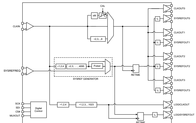
方框图
