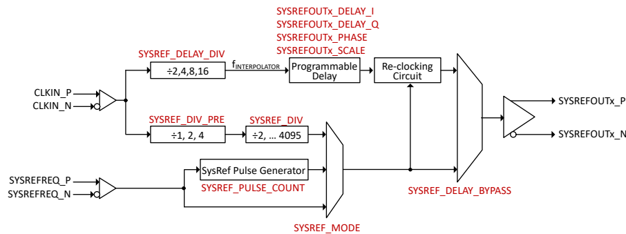
图 7-4. SYSREF Generator Diagram
