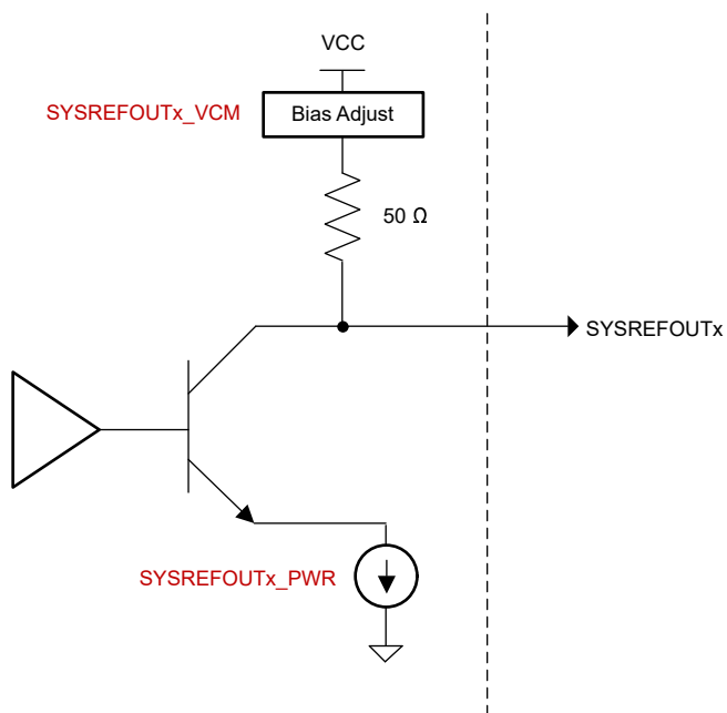
图 7-3. SYSREF Output Buffer
