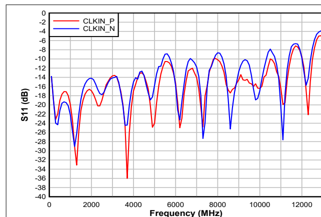
图 6-30. CLKIN S11 Magnitude
