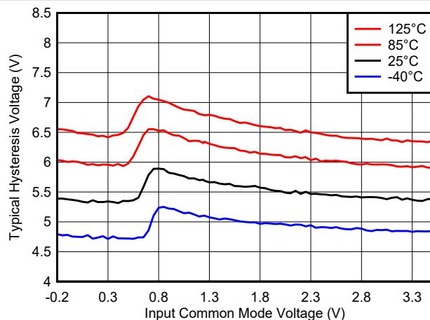
图 8-23. 迟滞电压与共模间的关系, 3.3V
