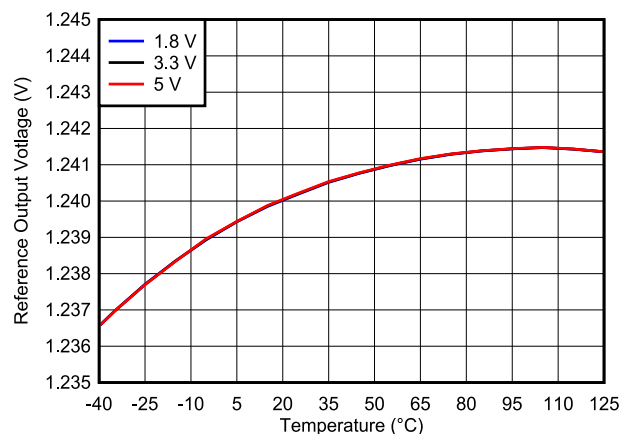
TLV3012B-Q1 基准电压与温度间的关系
