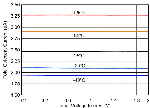
图 8-10. 电源电流与共模间的关系 - 1.8V
