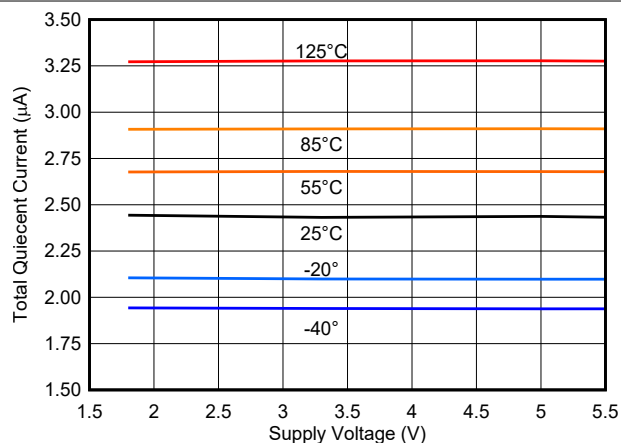
图 8-8. 电源电流与电源电压间的关系
