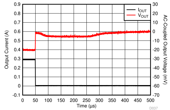
图 6-56. Load Transient
