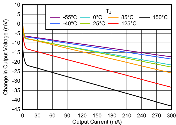
图 6-9. Load Regulation vs I_{OUT}
