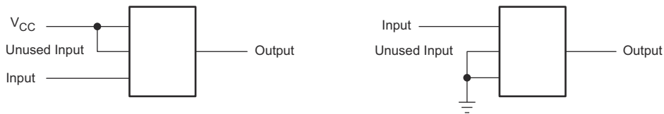
图 9-3. 布局图
