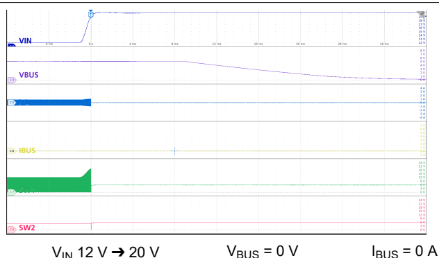
图 10-29. V_{IN(OVP)} Showing V_{BUS} Discharge
