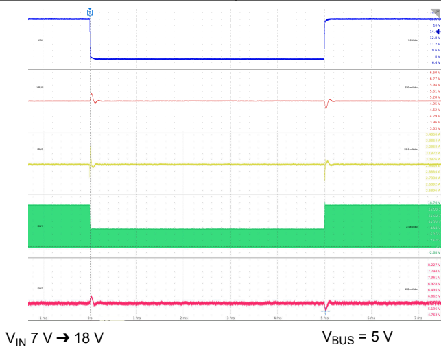
图 10-38. Line Transient: V_{BUS} = 5\text{ V}
