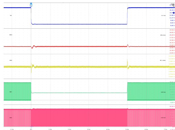
图 10-36. Line Transient: V_{BUS} = 15\text{ V}
