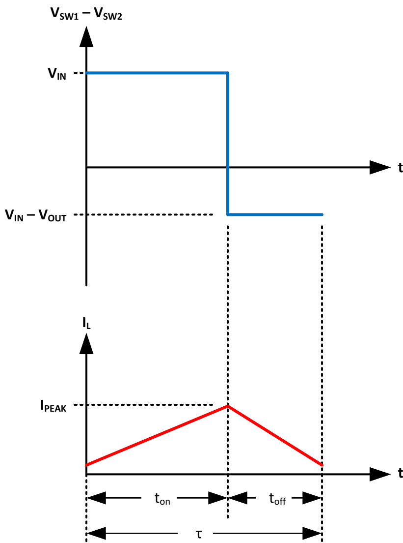
图 9-11. Boost State
