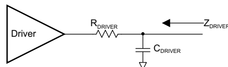
图 9-24. ZDRIVER Circuit
