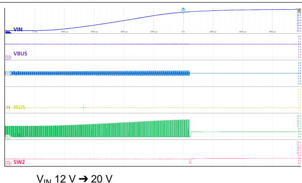
图 10-27. V_{IN(OVP)} Entry
