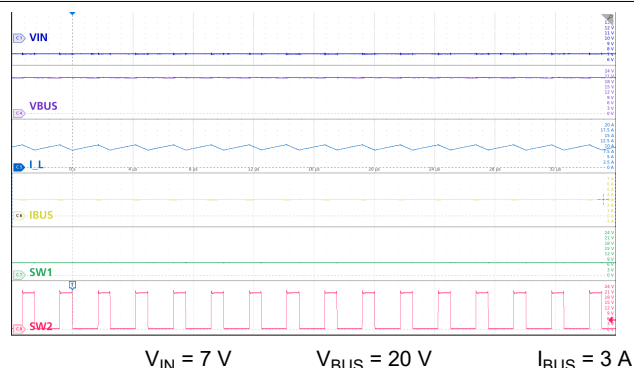
图 10-16. Boost Mode: Low V_{IN} , 3 A Load
