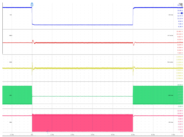
图 10-37. Line Transient: V_{BUS} = 9\text{ V}
