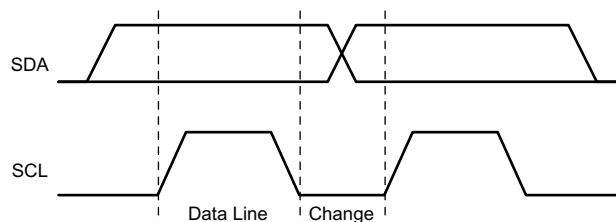
图 9-36. I²C Bit Transfer
