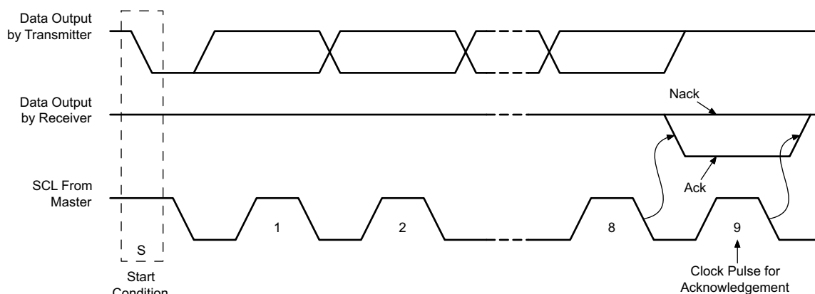
图 9-37. I²C Acknowledgment
