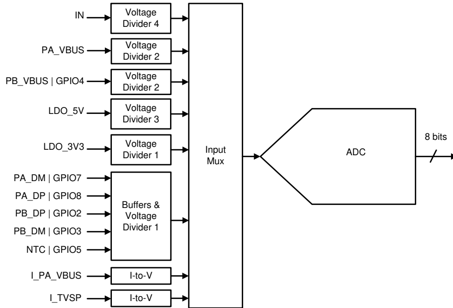
图 9-30. SAR ADC
