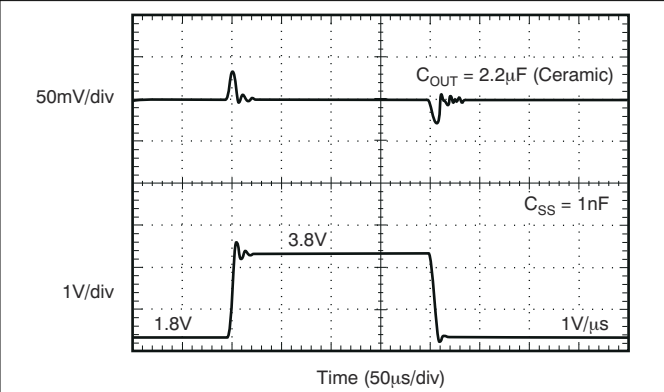
图 6-18. V_{IN} Line Transient
