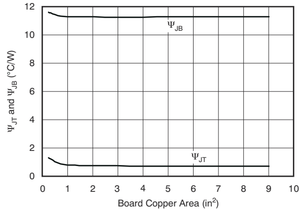
图 8-8. \Psi_{JT} 和 \Psi_{JB} vs Board Size
