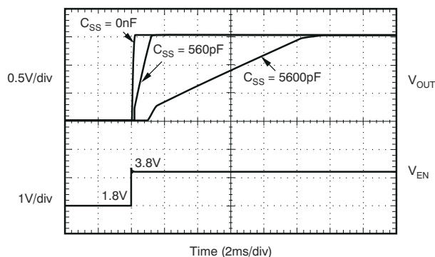
导通响应
