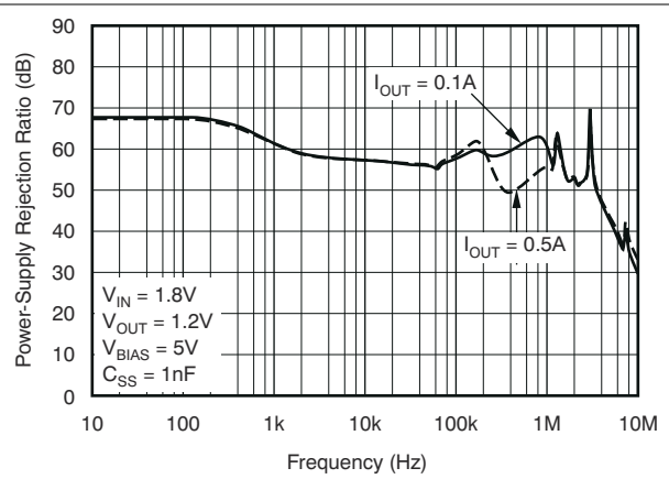
图 6-8. V_{BIAS} PSRR vs Frequency
