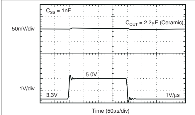
图 6-17. V_{BIAS} Line Transient
