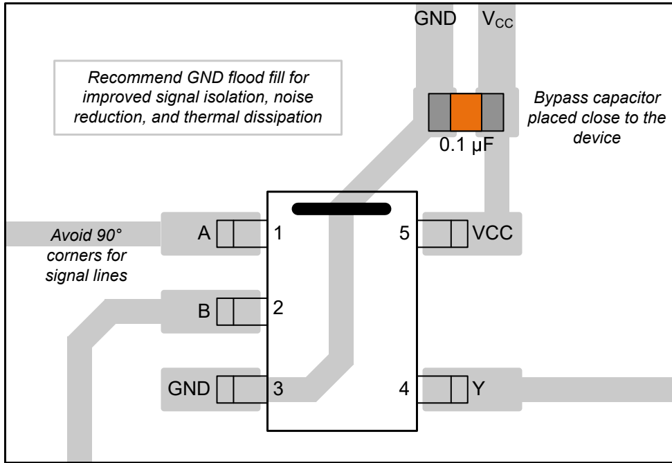
图 9-3. SN74LV1T08-Q1 的示例布局
