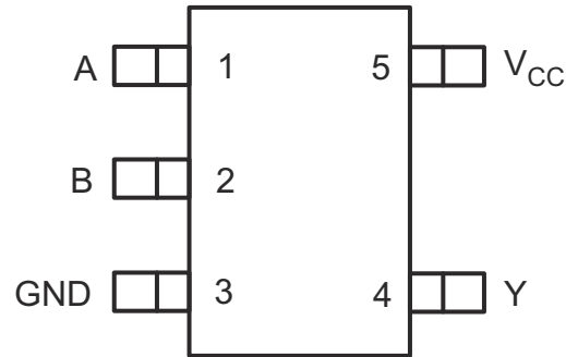
图 5-1. SN74LV1T08-Q1 DCK Package, 5-Pin SC-70 (Top View)
