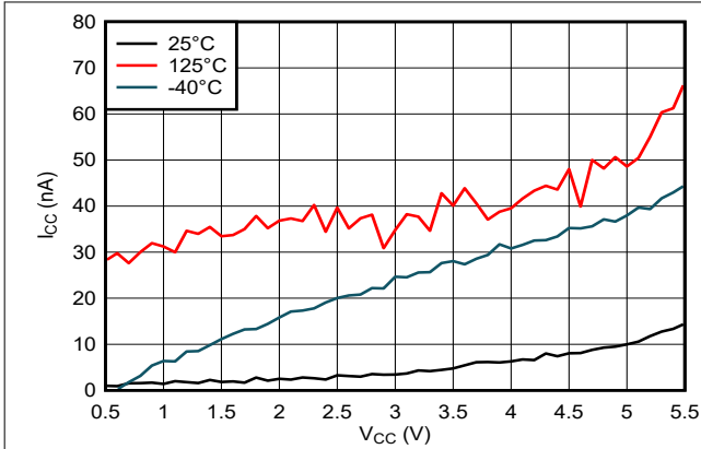
图 6-3. 电源电压两端的电源电流
