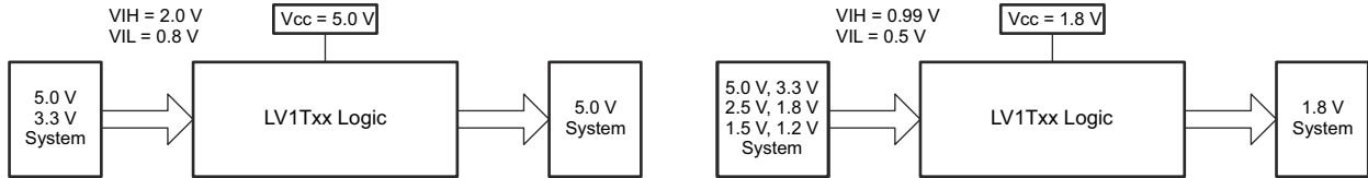
图 8-2. LV1Txx 升压和降压转换示例
